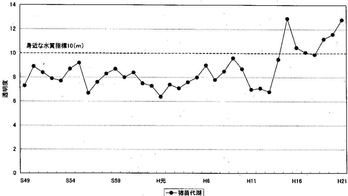
猪苗代湖の透明度(年平均値)の経年変化
