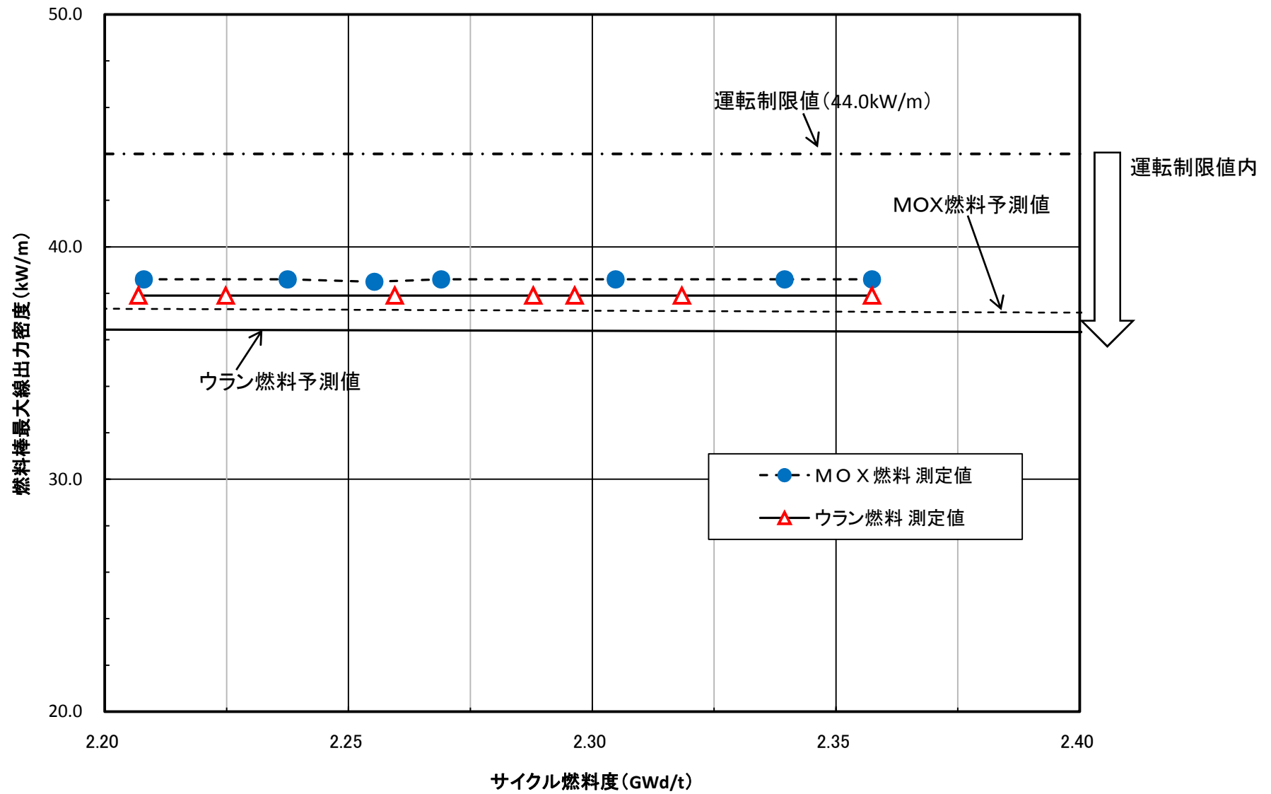
図2 燃料棒最大線出力密度の推移
