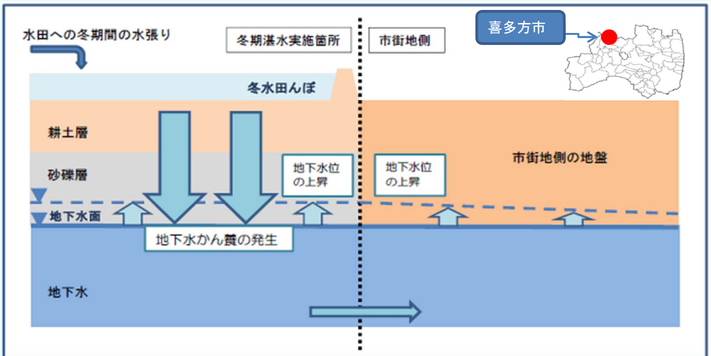
湛水開始直後の状況(平成26年11月8日)
