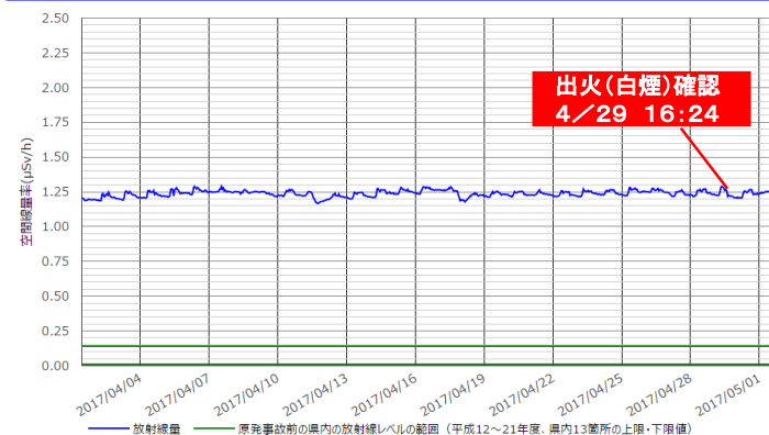
放射線モニタリングポスト 大熊町 野上一区地区集会所 4/29 16:00 1.23μSv/h → 5/1 12:00 1.24μSv/h
