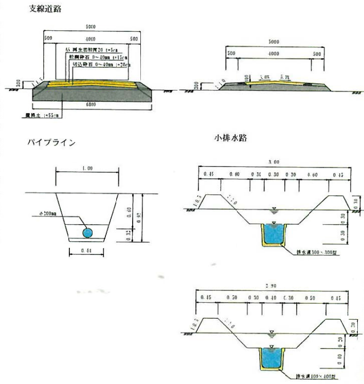
標準構造図
