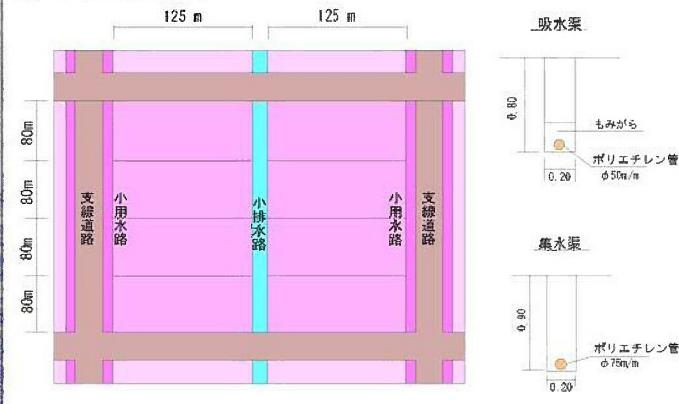
標準構造図
