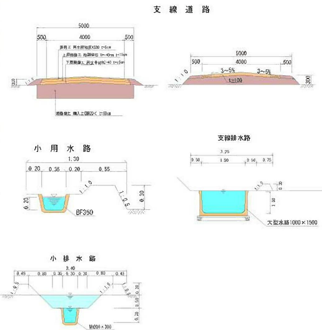
標準構造図
