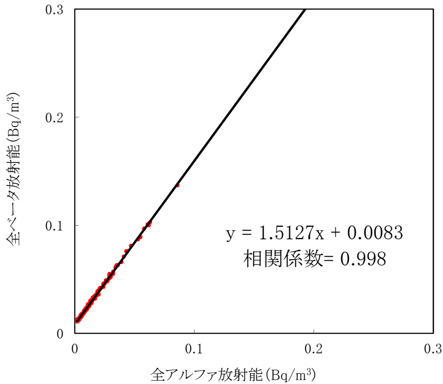
大気浮遊じんの全アルファ・全ベータ放射能の相関図 (MP-1) (平成31年1月～3月)
