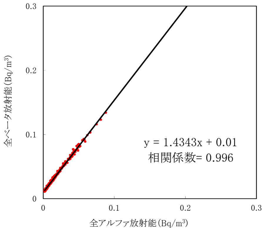
大気浮遊じんの全アルファ・全ベータ放射能の相関図 (MP-7) (平成31年1月～3月)
