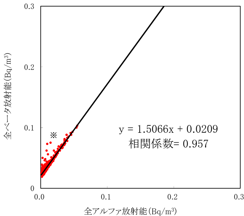
大気浮遊じんの全アルファ・全ベータ放射能の相関図 (MP-8) (平成31年1月～3月)
