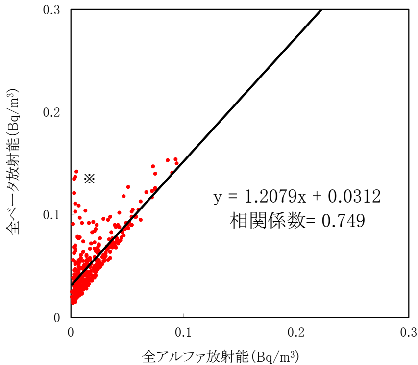
大気浮遊じんの全アルファ・全ベータ放射能の相関図 (MP-3) (平成31年1月～3月)
