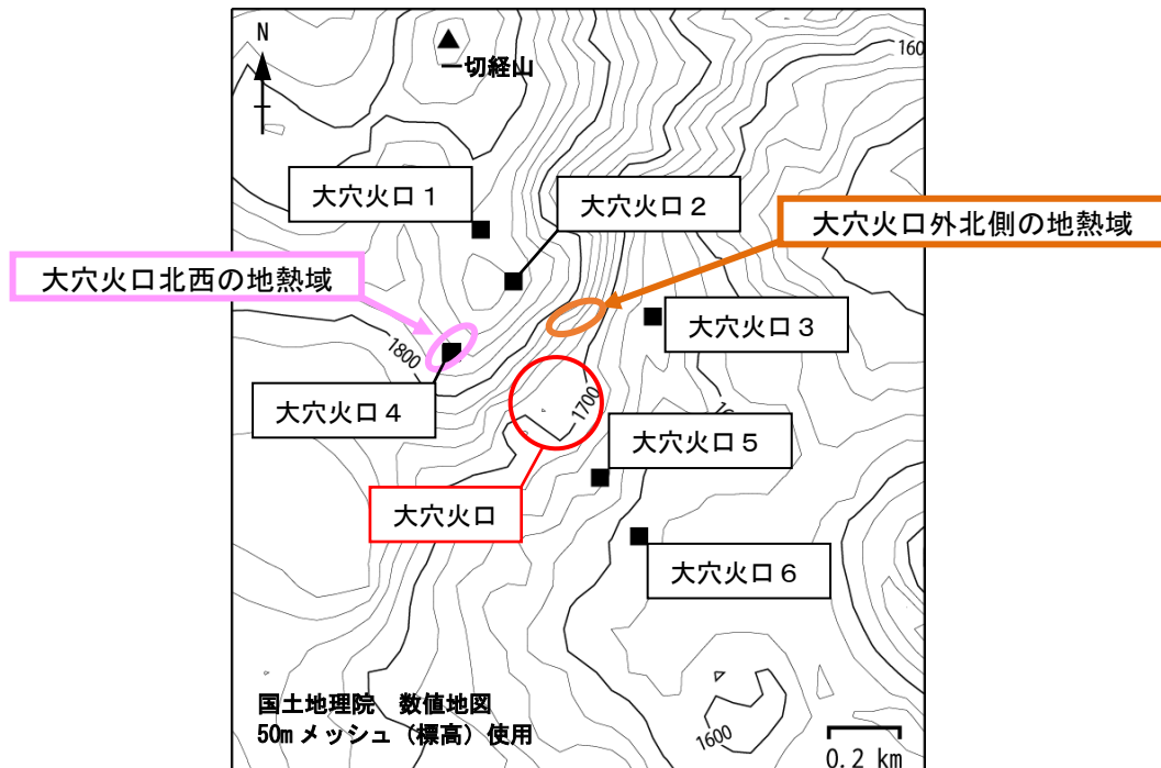
図16 吾妻山 全磁力観測点配置図
