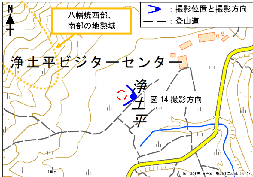
図13 吾妻山 浄土平周辺の状況
