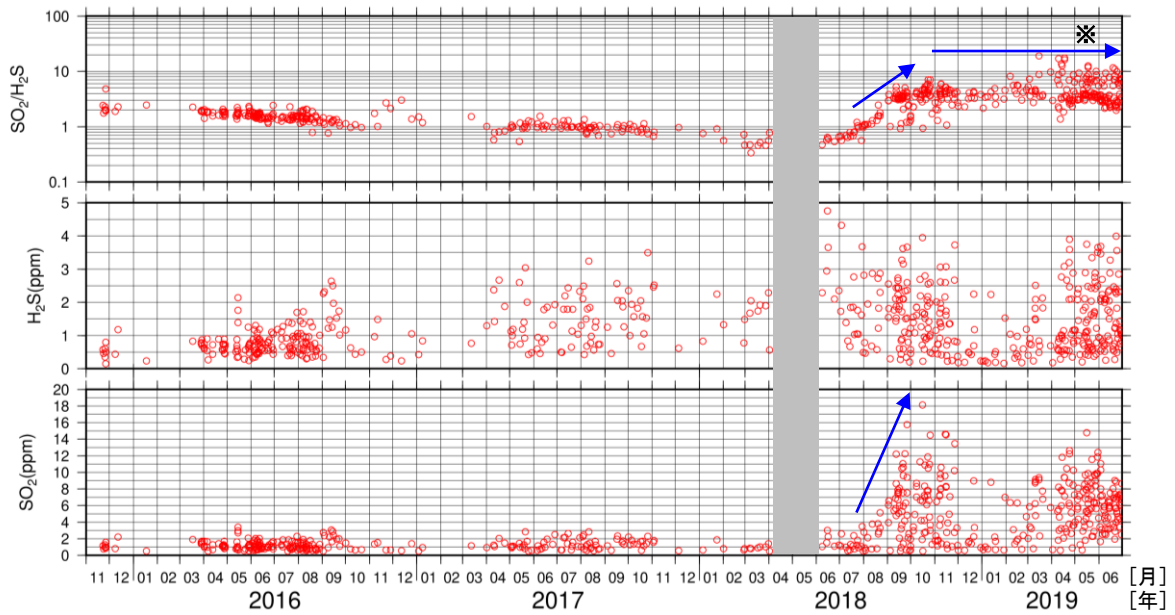
図15 吾妻山 火山ガス観測装置による観測（2015年11月～2019年6月）
