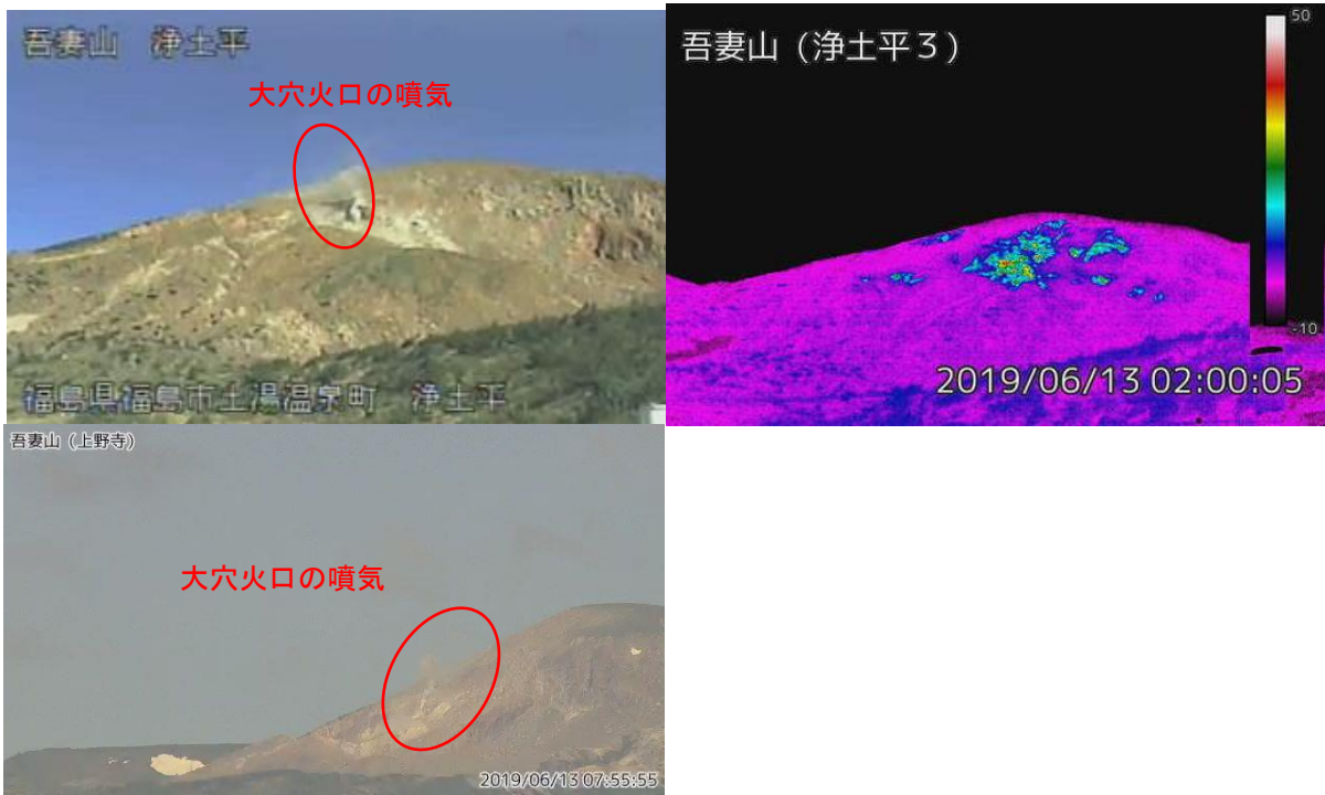
図10 吾妻山 大穴火口周辺の噴気の状態及び地表面温度分布（6月13日）
