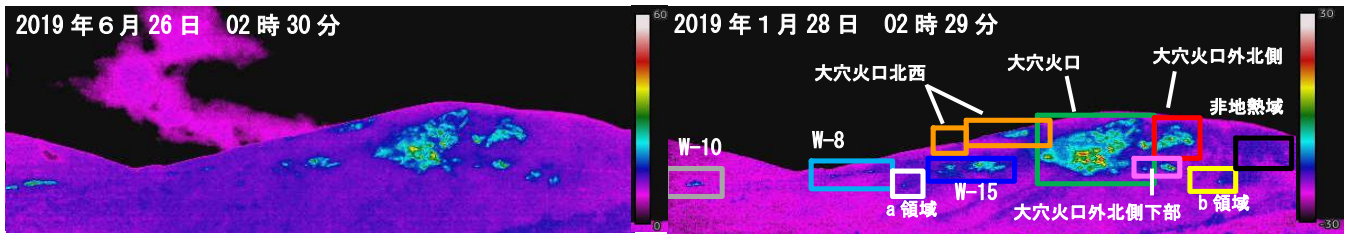
図8 吾妻山 浄土平3監視カメラ（熱映像）による大穴火口周辺の地熱域の状況
