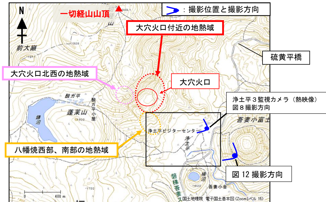
図11 吾妻山 大穴火口周辺の噴気と地熱域の分布及び写真と地表面温度分布撮影方向
