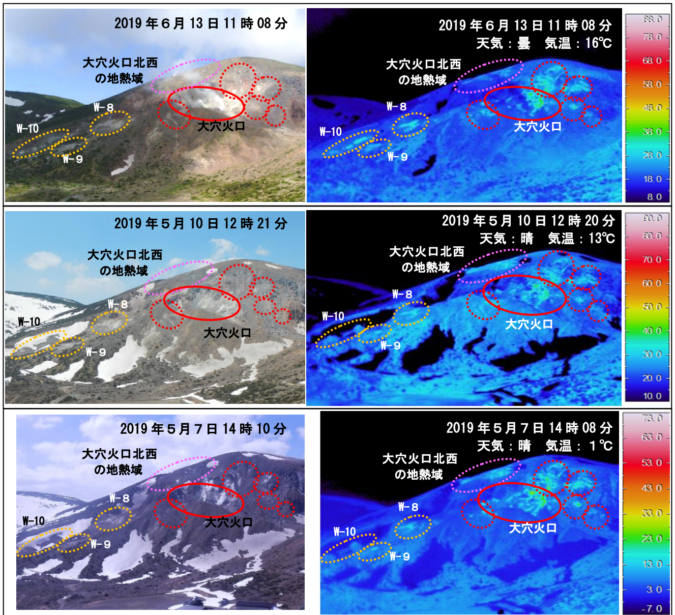
図 12 吾妻山 大穴火口付近及びその周辺の状況（左）と地表面温度分布（右）
