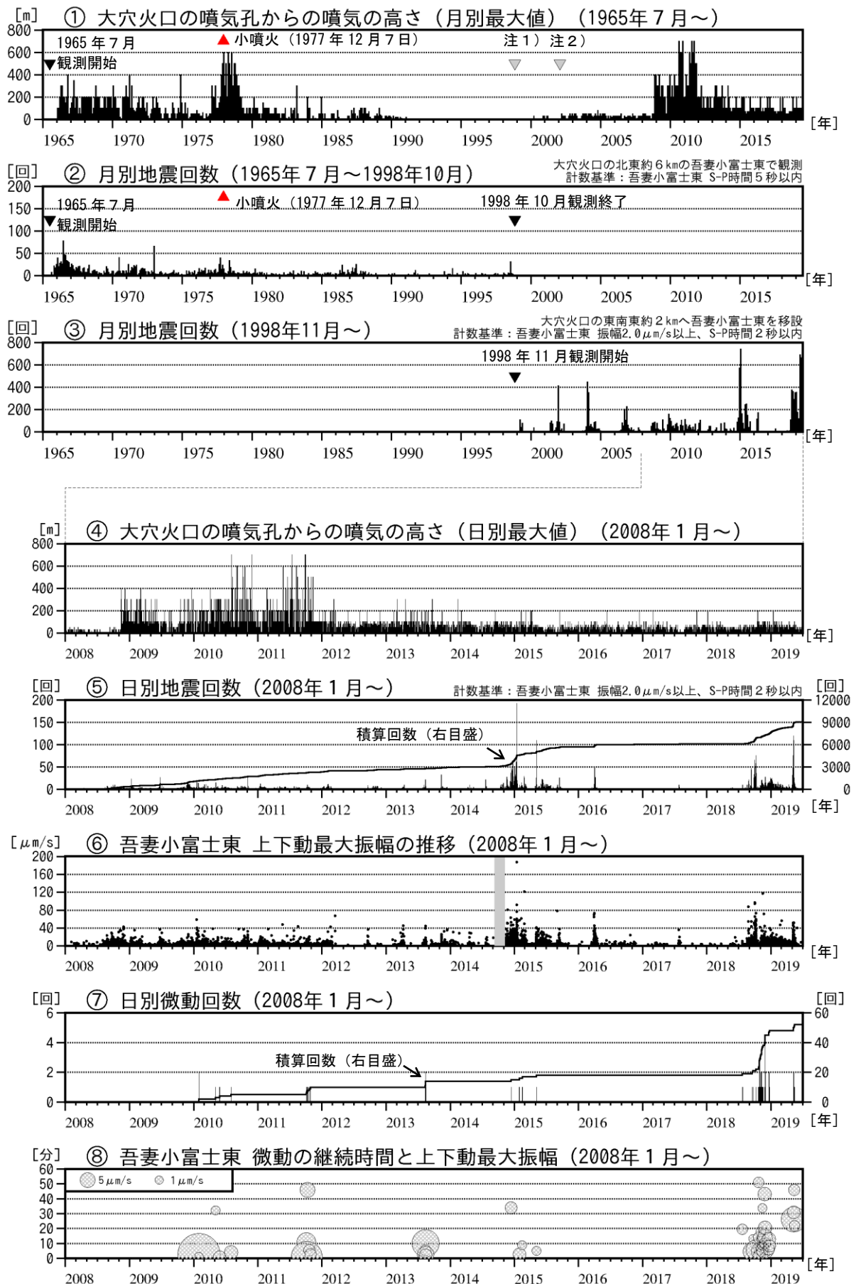
図4 吾妻山 火山活動経過図（1965年7月～2019年6月）
