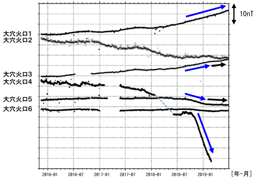
図17 吾妻山 全磁力連続観測点の全磁力値変化（2015年11月～2019年6月）
