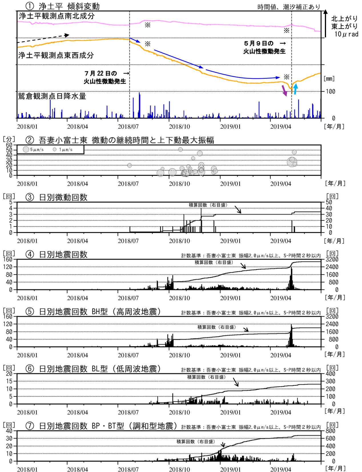
図2 吾妻山 浄土平観測点における傾斜変動、火山性微動の発生状況及び日別地震回数 (2018年1月～2019年6月)
