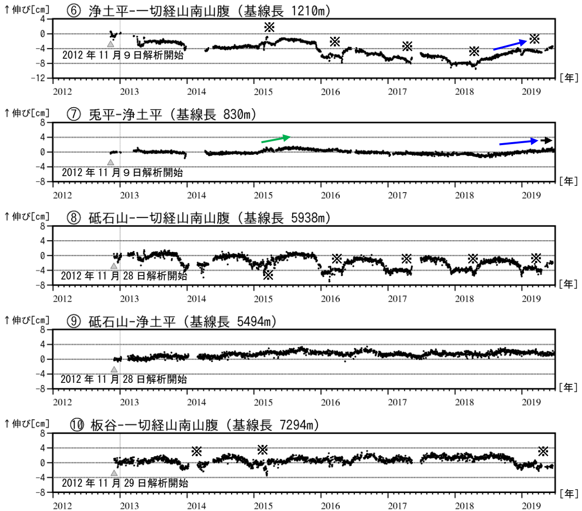
図6 吾妻山 GNSS 基線長変化図（2012年11月～2019年6月）
