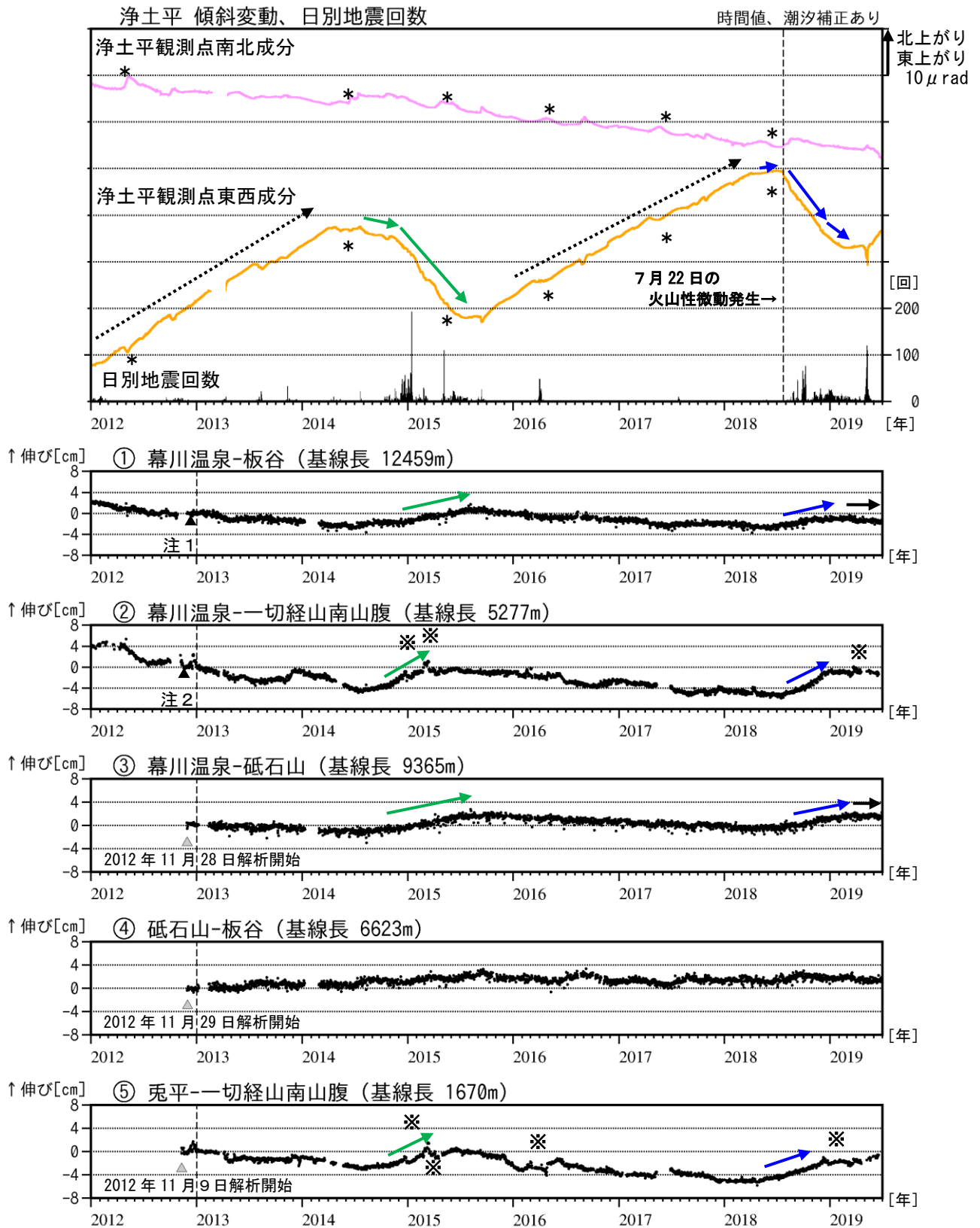
図5 吾妻山 傾斜変動及びGNSS基線長変化図（2012年1月～2019年6月）
