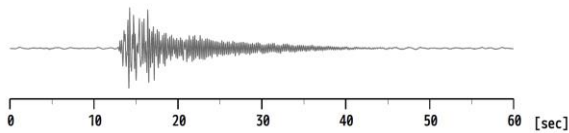
図1 吾妻山 主な火山性地震の特徴と波形例
