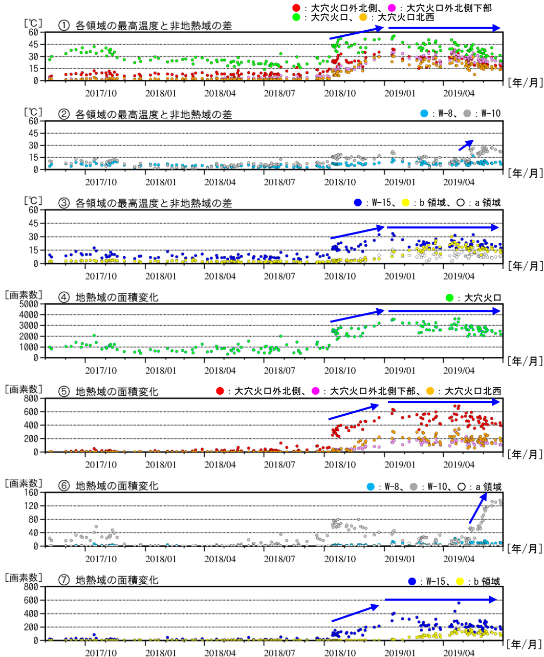
図9 吾妻山 監視カメラによる大穴火口周辺の地熱域の経過（2017年8月～2019年6月）
