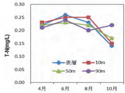
図 4 T-N の季節変動
