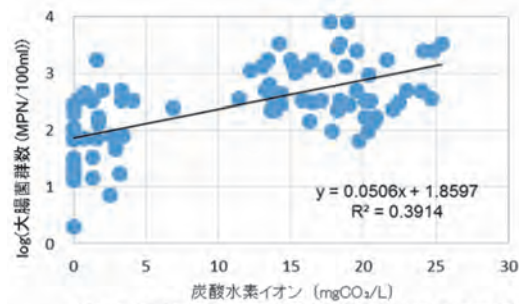
図41 炭酸水素イオンと大腸菌群数(2011～2017年)
