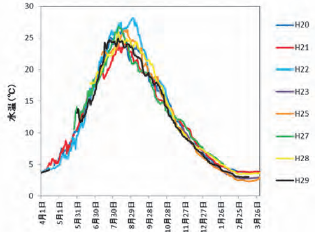
図 5 水深 5m の水温変化 (H20~H29)
