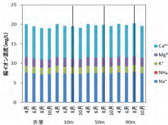
図 6 陽イオン成分の水深別季節変動
