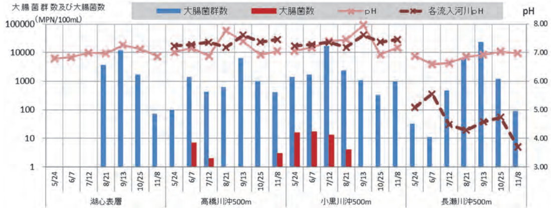
図 16 各河川沖 500m 地点等の pH の推移
