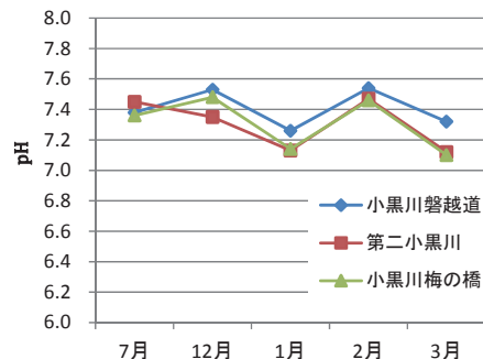
図 5 小黒川の pH 推移
