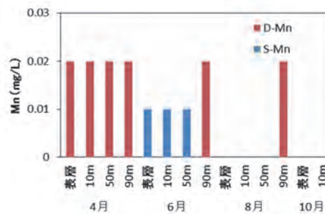
図 10 Mn の季節変動
