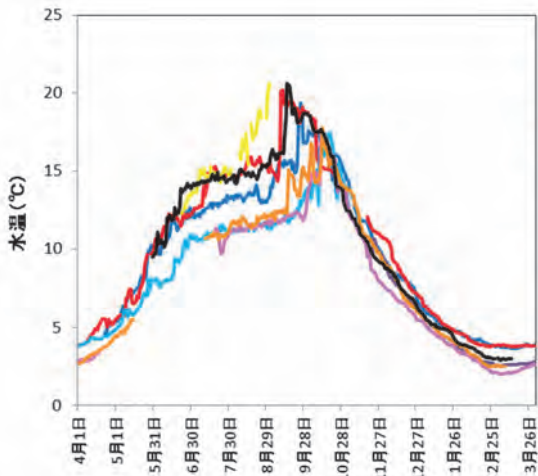
図 6 水深 15m の水温変化 (H20~H29)
