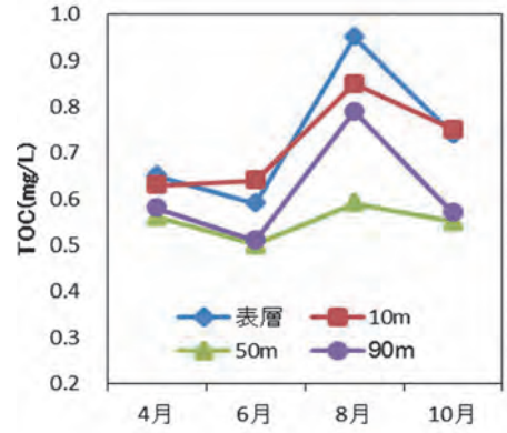
図12 TOCの季節変動
