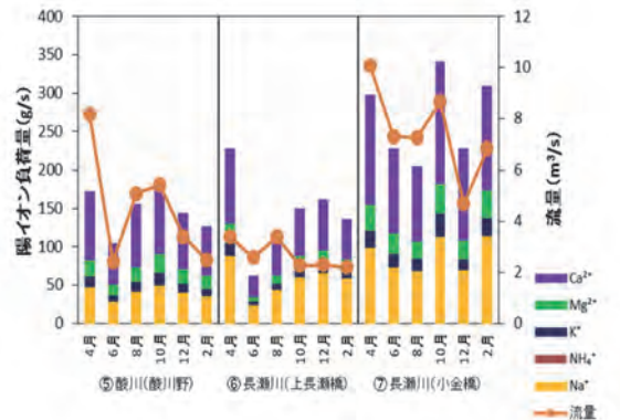
図 25-2 下流域河川の陽イオン負荷量の季節変動
