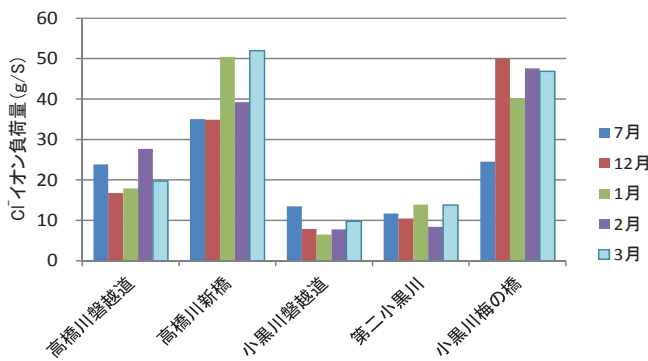
図 25 高橋川、小黒川の Cl - イオン負荷量
