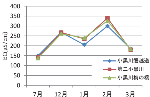
図9 小黒川のEC推移
