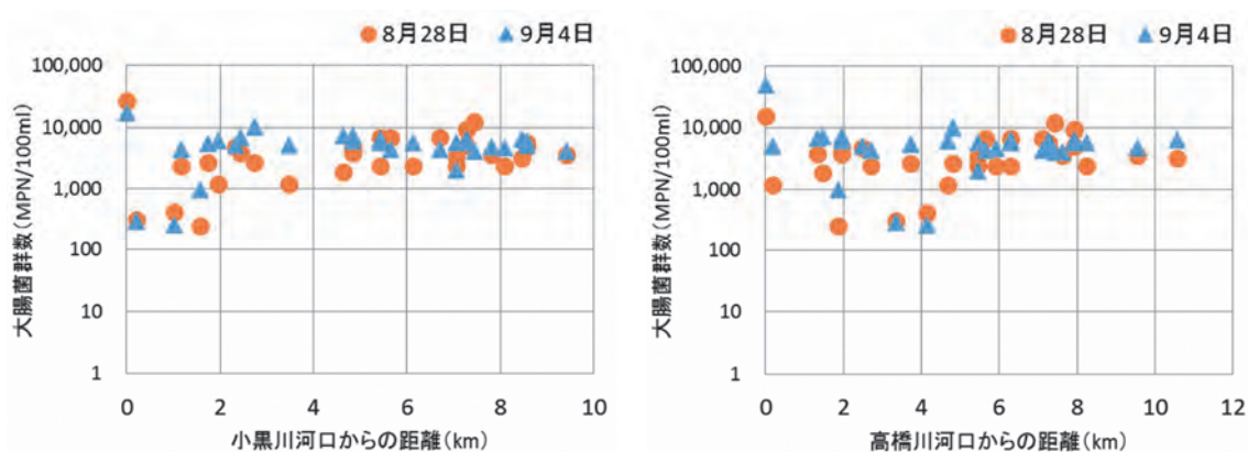
図 7 小黒川梅の橋及び高橋川新橋と湖北部 (No.1~29) の各河口からの距離と大腸菌群数の調査結果 (小黒川梅の橋及び高橋川新橋の結果は、河口からの距離を「0」とした)
