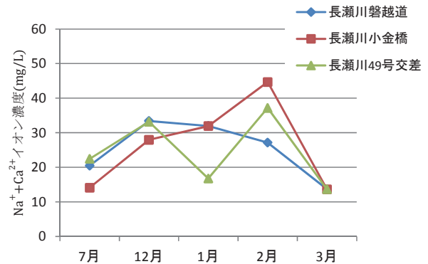
図18 長瀬川のNa + +Ca 2+ イオン濃度推移
