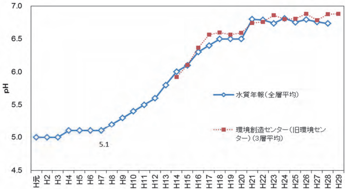
図13 pH経年変化
