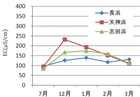
図7 猪苗代湖3浜のEC推移
