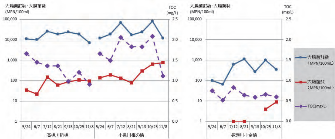
図 14 各河川の大腸菌群と TOC 等の推移
