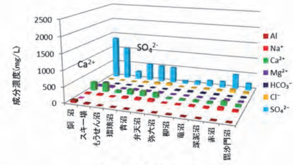
図8 主要成分濃度 2016年
