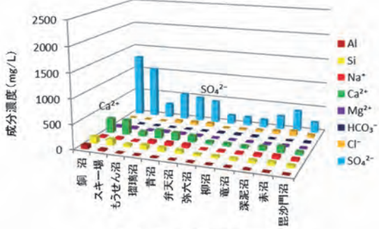
図4 主要成分濃度 2012年
