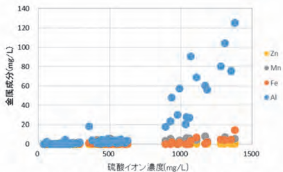
図34 金属成分濃度と硫酸イオン濃度(2011~2017年)
