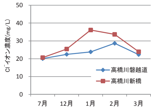
図20 高橋川のCl⁻イオン濃度推移
