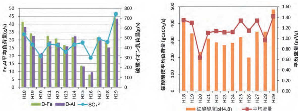
図 28 ③ 高森川(酸川合流前)の酸性成分負荷量及び流量の経年変化
