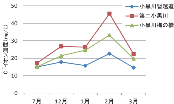
図21 小黒川のCl⁻イオン濃度推移
