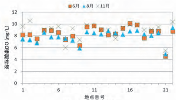
図13 DOの季節変動
