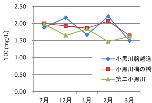
図 29 小黒川の TOC 推移
