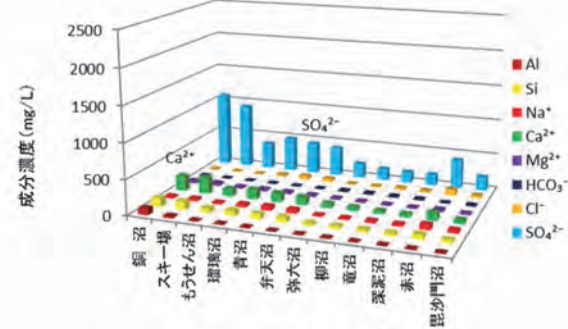
図7 主要成分濃度 2015年
