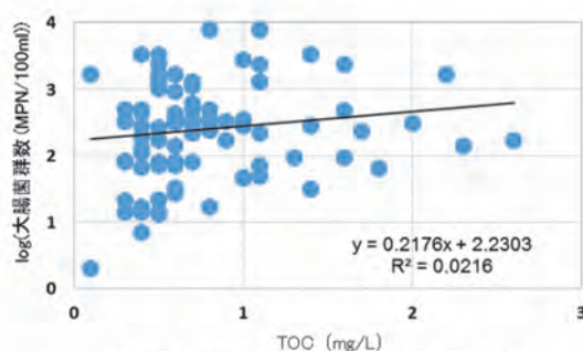
図39 TOCと大腸菌群数(2011～2017年)
