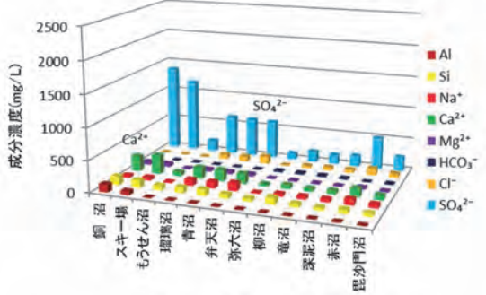
図3 主要成分濃度 2011年
