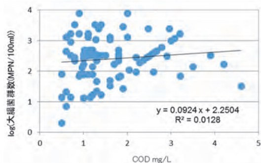
図38 CODと大腸菌群数(2011～2017年)
