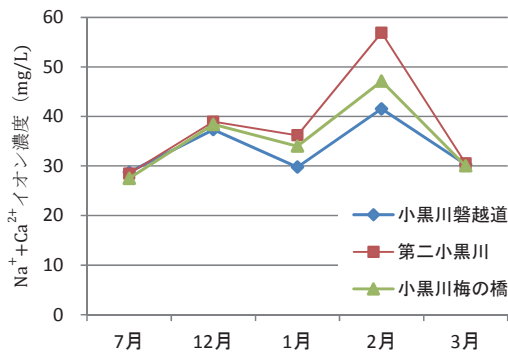
図17 小黒川のNa + +Ca 2+ イオン濃度推移
