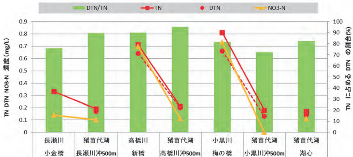
図3 T-N等の濃度及び溶存態の割合
