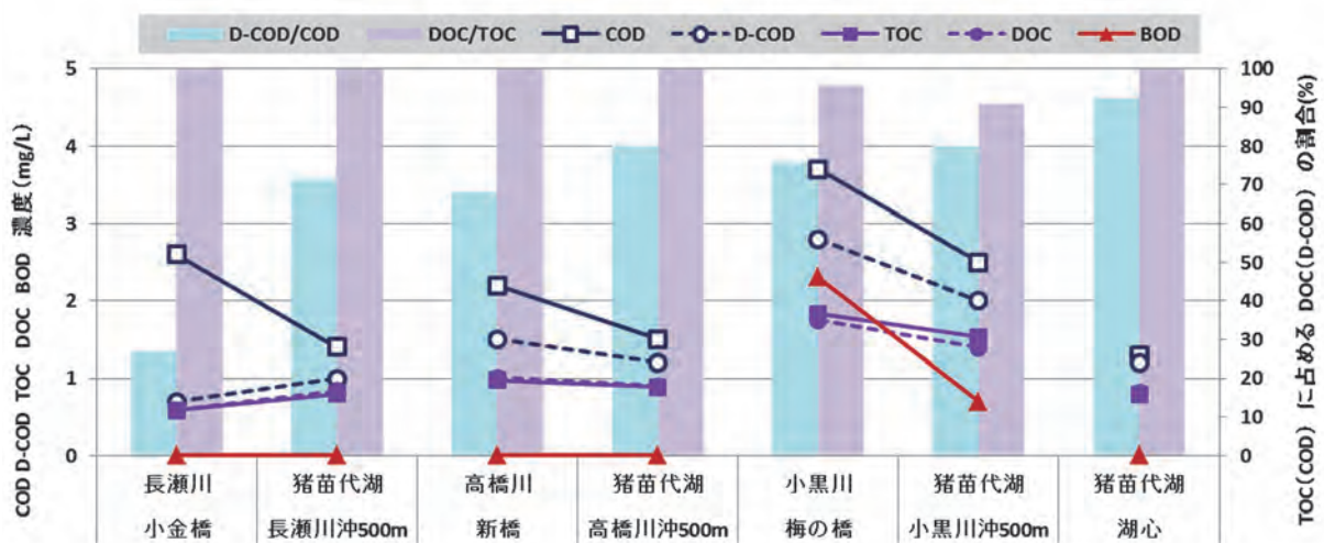
図2 各地点におけるCOD、TOC等濃度及び溶存態の割合
