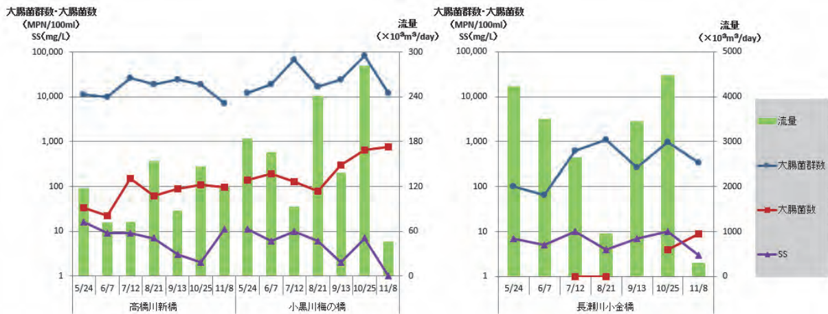
図 12 各河川の流量と SS 等の推移
