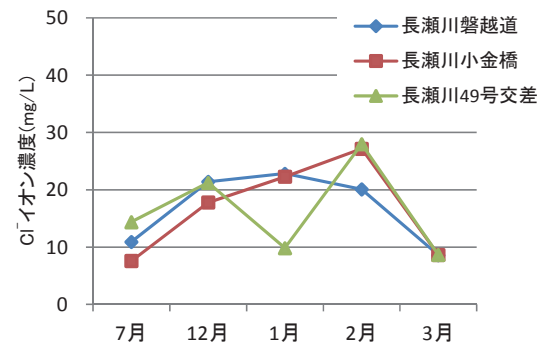
図22 長瀬川のCl⁻イオン濃度推移
