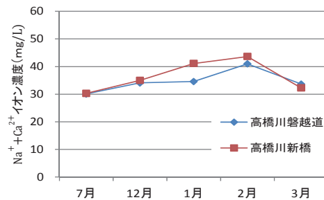
図16 高橋川のNa + +Ca 2+ イオン濃度推移
