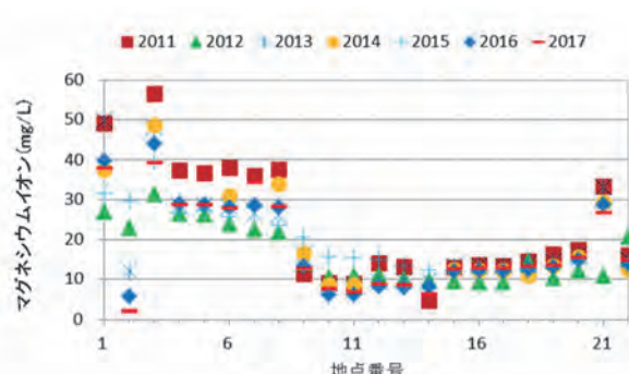
図26 マグネシウムイオン
