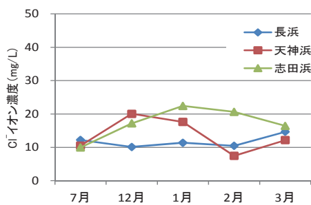
図19 猪苗代湖3浜のCl⁻イオン濃度推移
