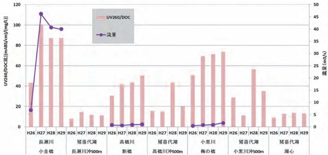
図6 平成26年度から平成29年度のUV260/DOC比及び流量
