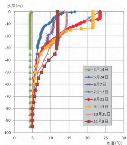
図3 湖心の鉛直分布
