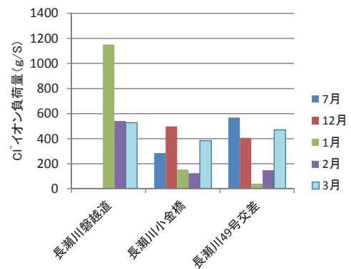
図 26 長瀬川の Cl - イオン負荷量
