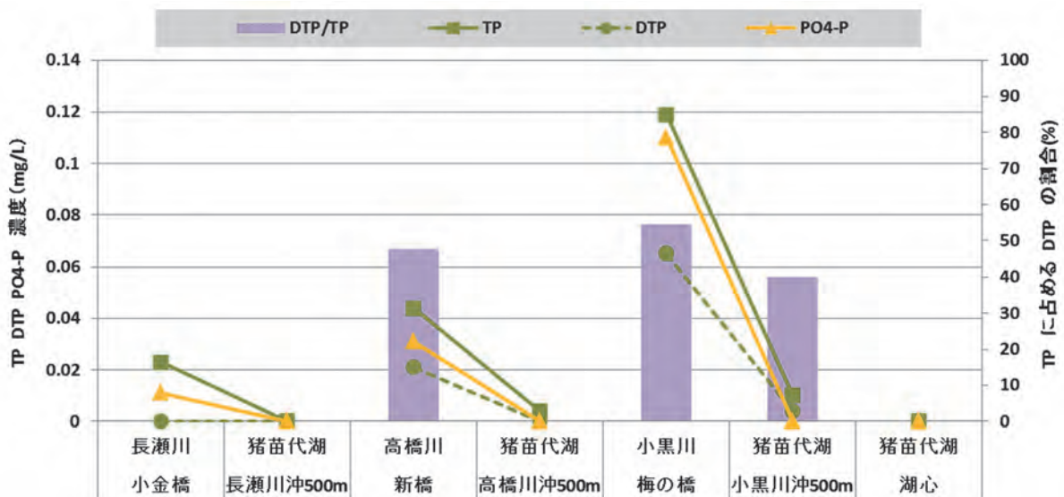
図4 T-P等の濃度及び溶存態の割合
