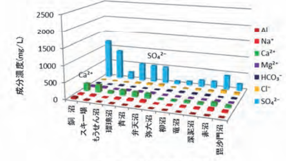
図9 主要成分濃度 2017年
