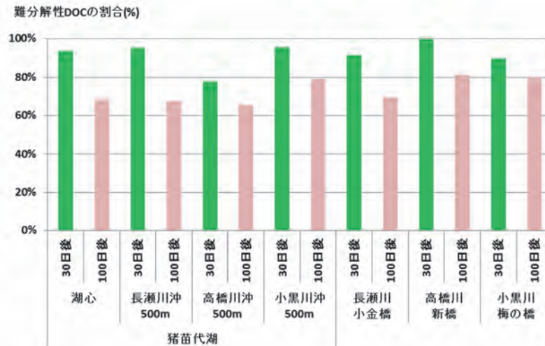
図8 生分解試験30日後の難分解性DOCの割合
