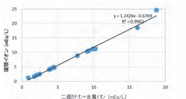
図24 硫酸イオン当量濃度と(金属+2価カチオン)イオン当量濃度との関係(2017年)
