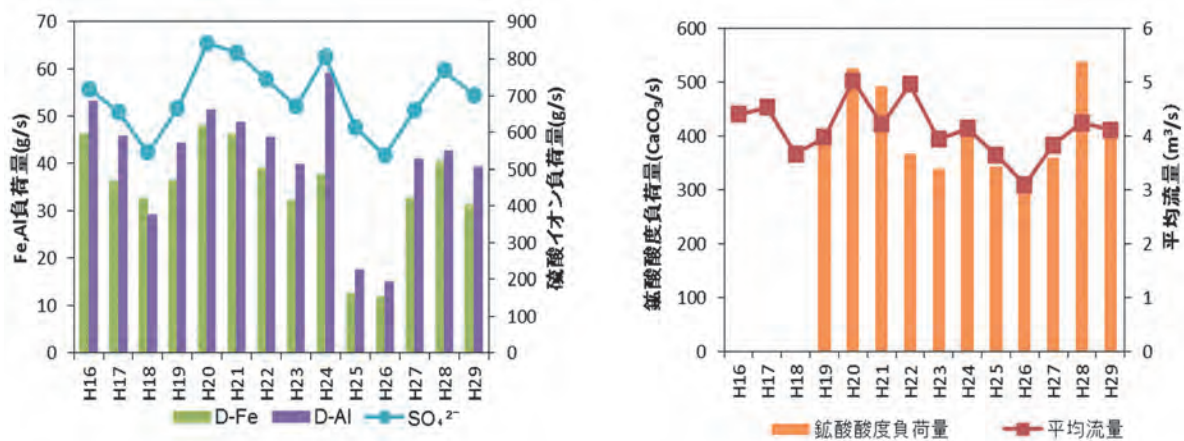
図 30 ⑤ 酸川(酸川野)の酸性成分負荷量及び流量の経年変化
