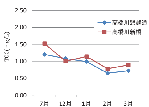
図 28 高橋川の TOC 推移
