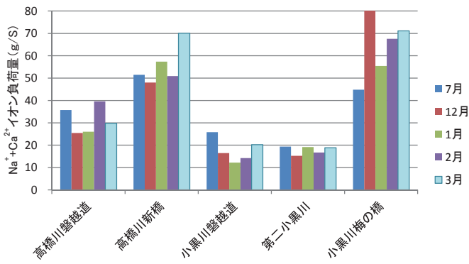
図 23 高橋川、小黒川の Na + +Ca 2+ イオン負荷量
