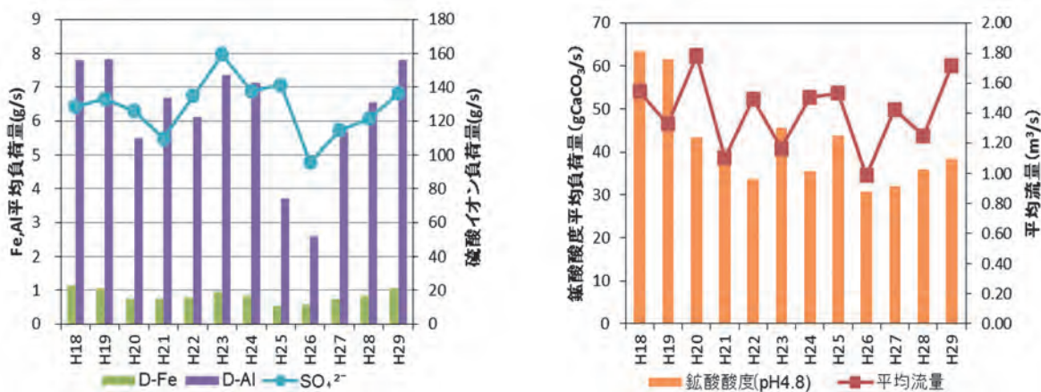
図 29 ④ 酸川(高森川合流前)の酸性成分負荷量及び流量の経年変化
