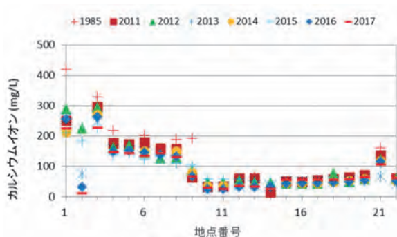
図25 カルシウムイオン
