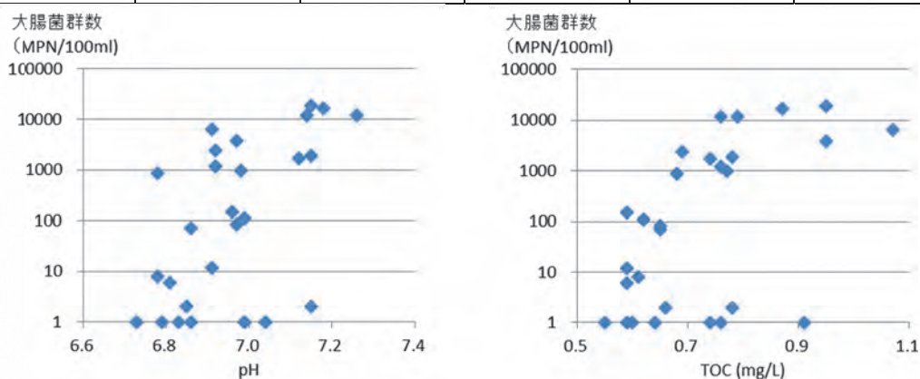
図8 湖心における大腸菌群数とpH及びTOCの相関関係
