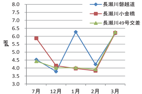
図 6 長瀬川の pH 推移
