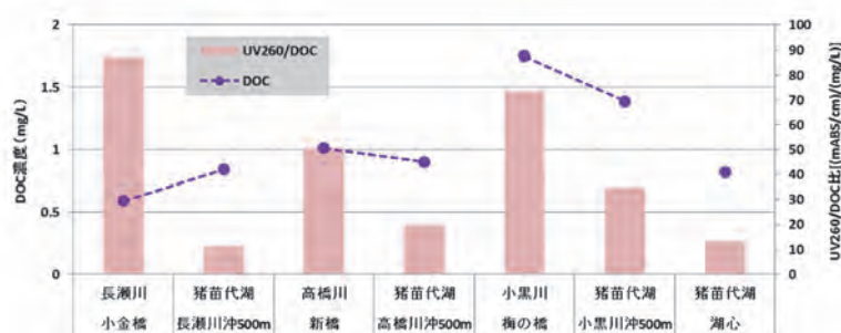
図 5 UV260/DOC 比及び DOC 濃度
