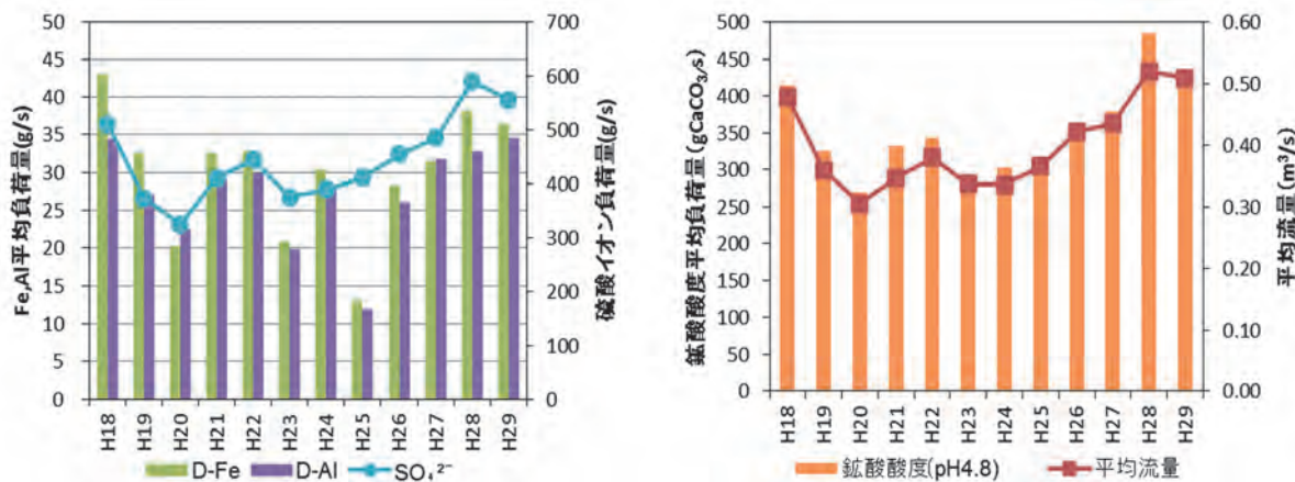
図 27 ② 硫黄川(高森川合流前)の酸性成分負荷量及び流量の経年変化
