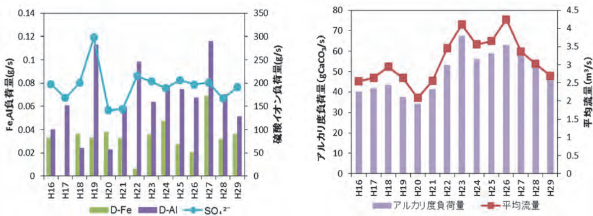
図 31 ⑥ 長瀬川(上長瀬橋)の酸性成分負荷量及びアルカリ度負荷量及び流量の経年変化
