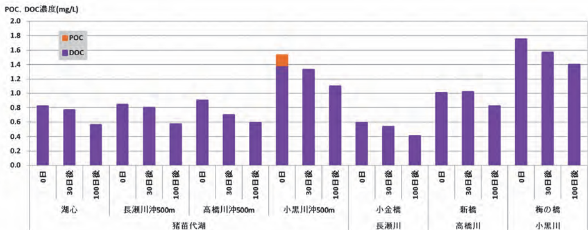
図7 生分解試験によるDOC等の変化
