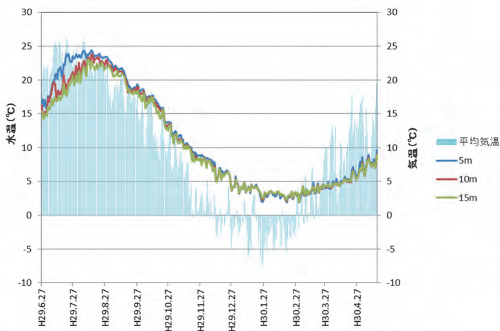
図 9 平成 29 年度における猪苗代湖長瀬川河口沖 300m の水深 5m 日平均水温及び日平均気温の関係
