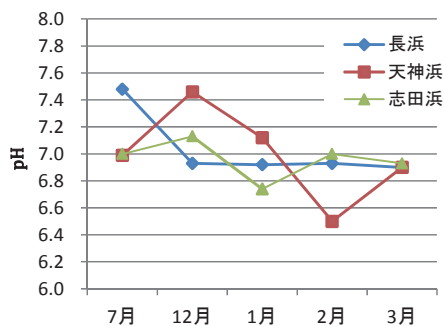
図 3 猪苗代湖 3 浜の pH 推移
