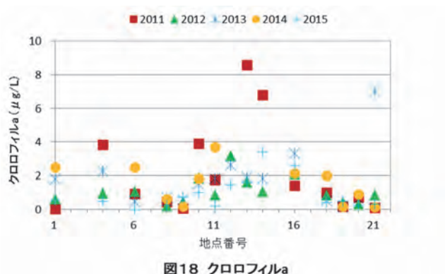
図18 クロロフィルa
