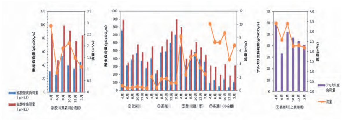
図 23 酸度負荷量及びアルカリ度負荷量の季節変動
