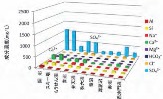
図6 主要成分濃度 2014年
