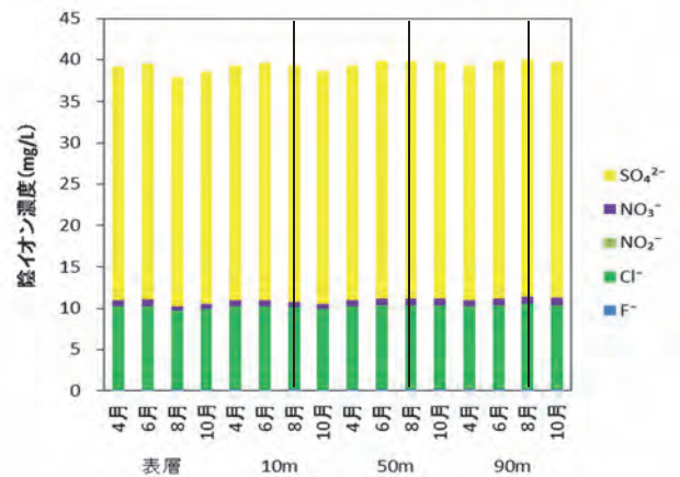
図 7 陰イオン成分の水深別季節変動
