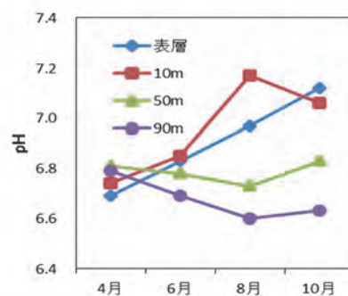
図 3 pH の季節変動
