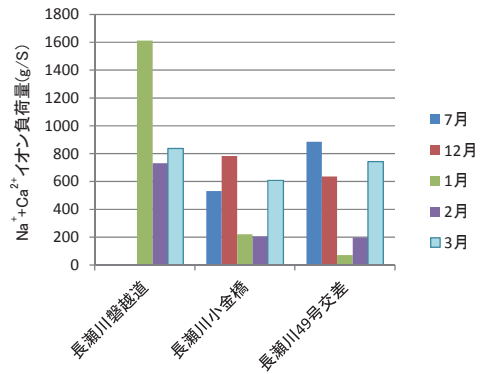
図 24 長瀬川の Na + +Ca 2+ イオン負荷量
