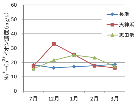
図15 猪苗代湖3浜のNa + +Ca 2+ イオン濃度推移
