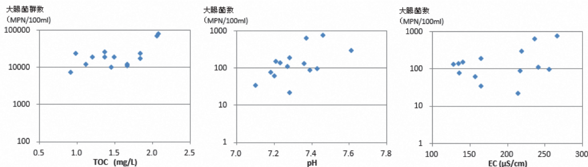
図 15 高橋川新橋及び小黒川梅の橋における各測定項目の相関関係
