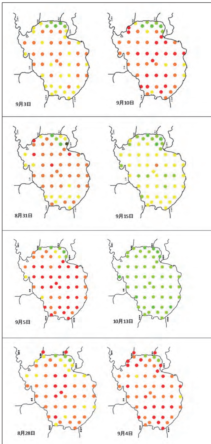
別図1 平成26～29年調査における猪苗代湖の大腸菌群数
