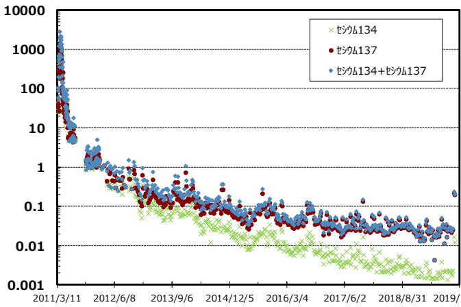
①福島第二 北放水口付近 (T-3) 海水セシウム濃度 (上層)
