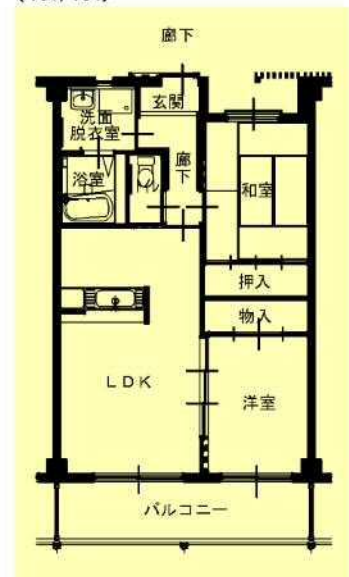
2LDK 高齢者仕様 (103, 104)
