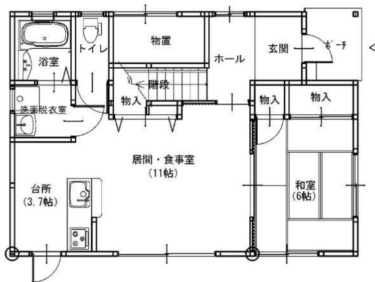
3LDK 1階
