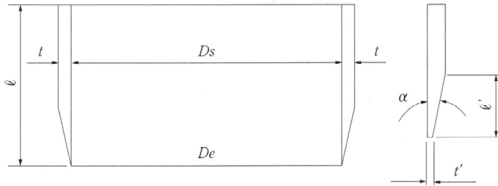
図 7-1 サンプリングチューブ
