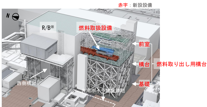
燃料取り出し用構台概念図（鳥瞰図）
