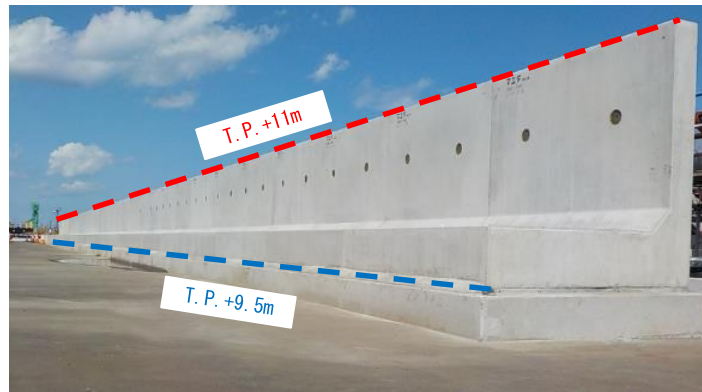
現地据付状況（2019年9月25日撮影）
