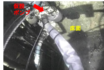
3号機T/B地下1階(最下階)の床面露出状況
