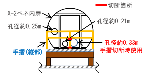
PCV内側から見た手摺切断範囲イメージ
