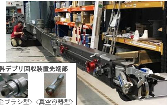
ロボットアーム
