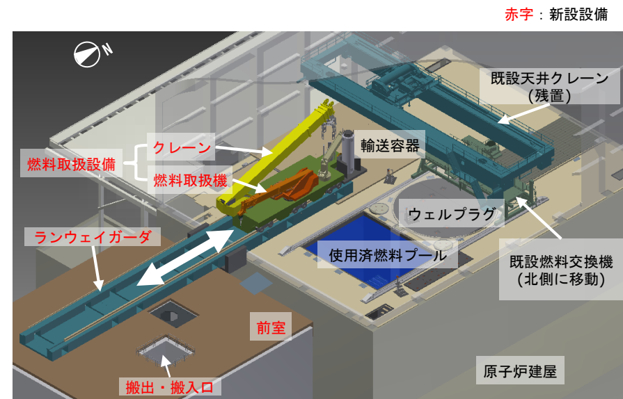
燃料取扱設備概念図（鳥瞰図）
