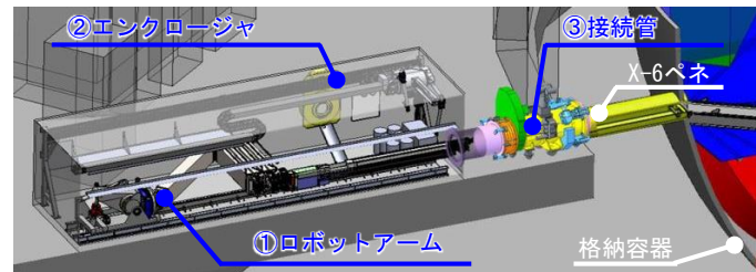
試験的取り出し装置の全体像
