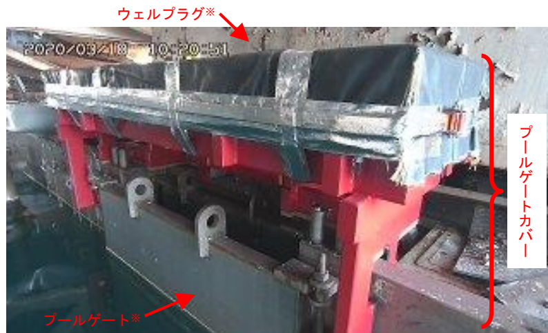
プールゲートカバーの設置状況
