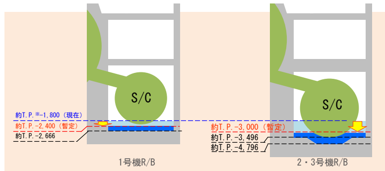
水位低下イメージ
