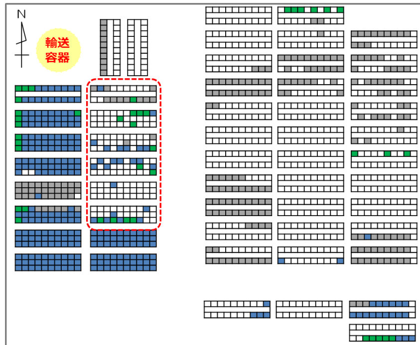
3号機使用済燃料プール (34回目までの取り出し状況を反映)
