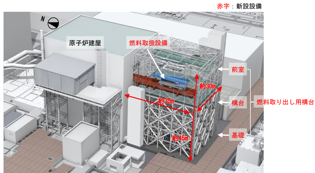
燃料取り出し用構台概念図（鳥瞰図）
