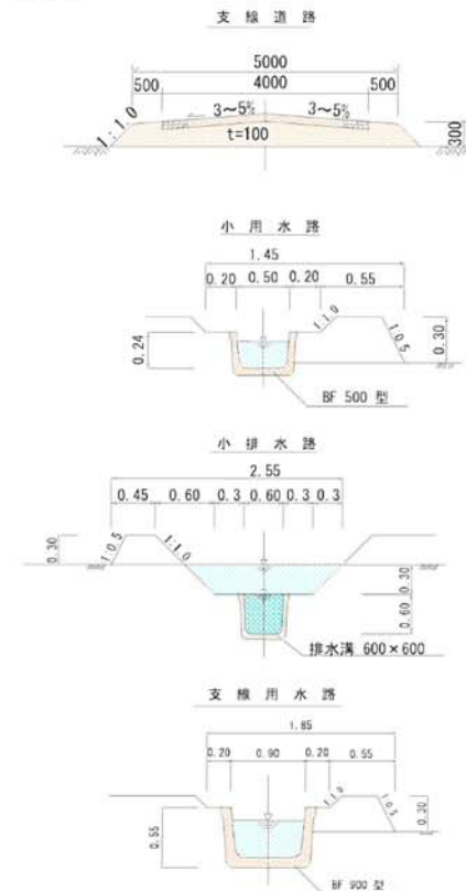
標準構造図
