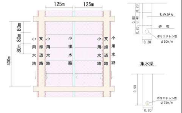
標準構造図
