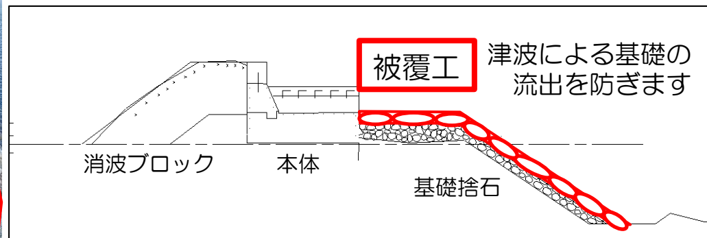
防波堤改良 L=262m
