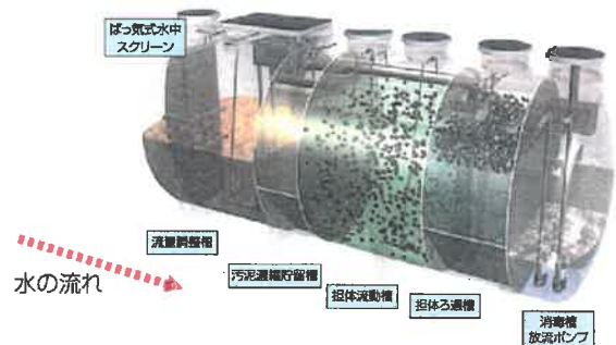
低コスト小型処理施設の完成イメージ
