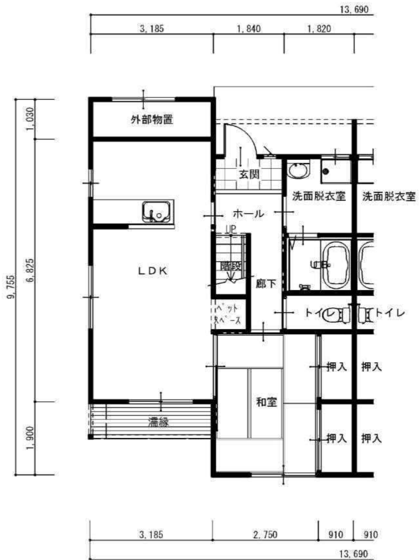
1階 平面図
