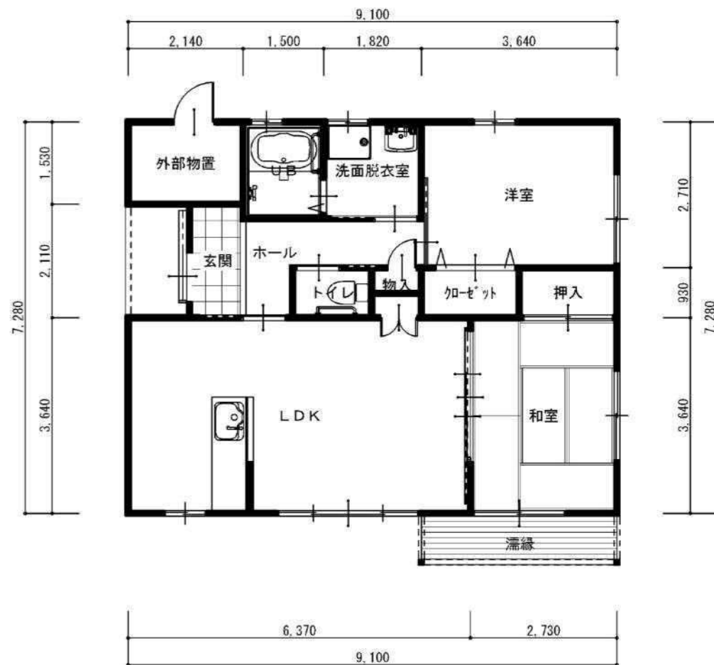
1階 平面図
