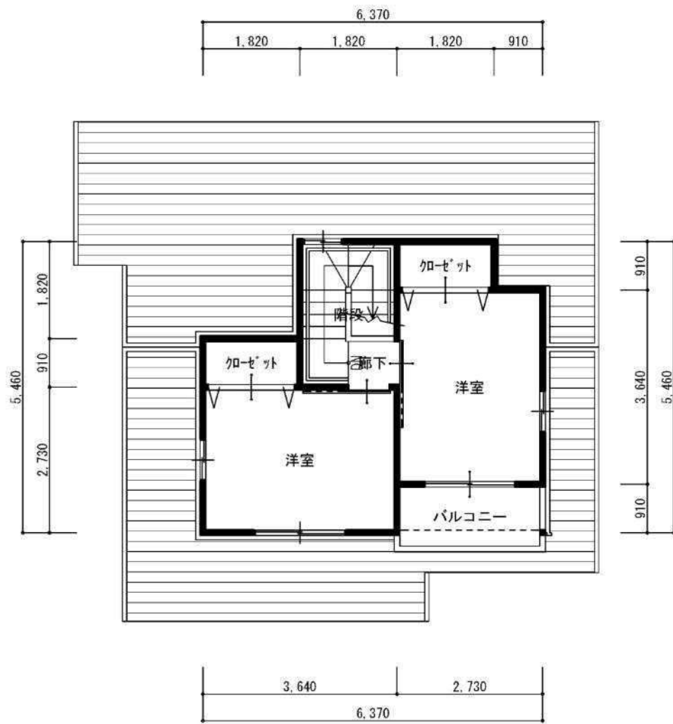
2階 平面図
