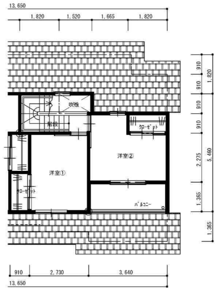
2階平面図
