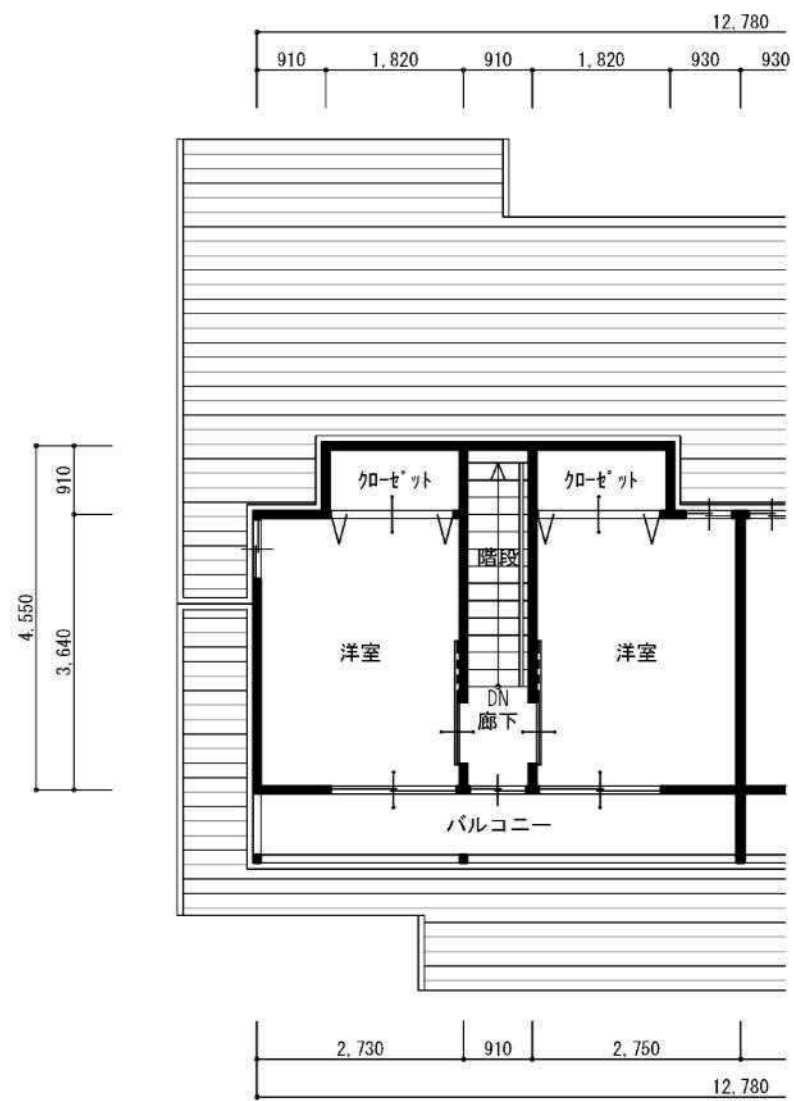
2階 平面図
