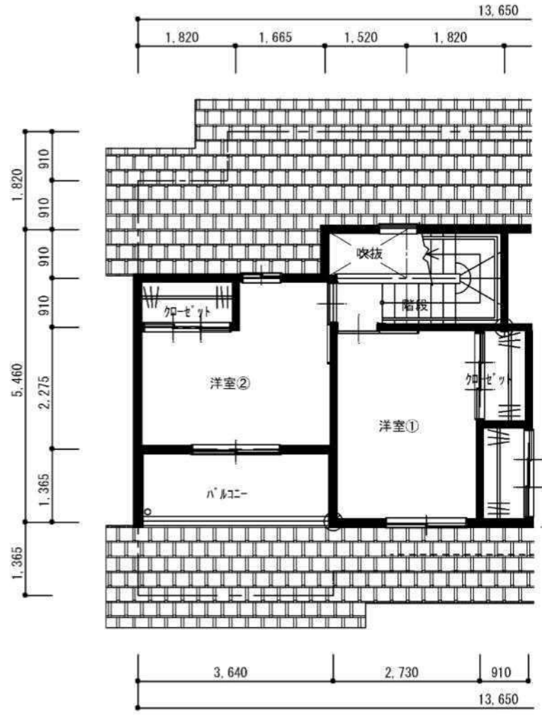
2階平面図
