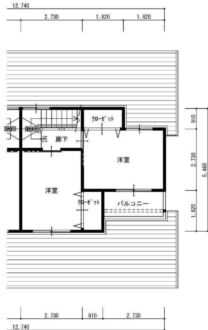
2階 平面図
