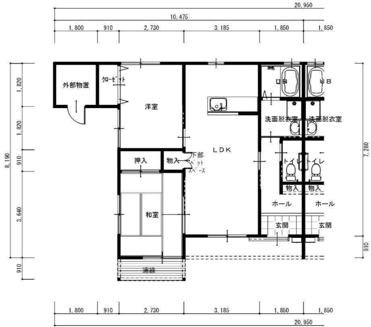
1階 平面図
