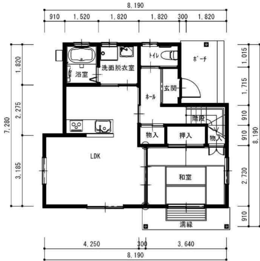
1階平面図
