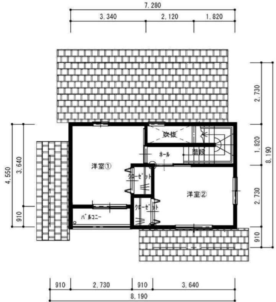
2階平面図
