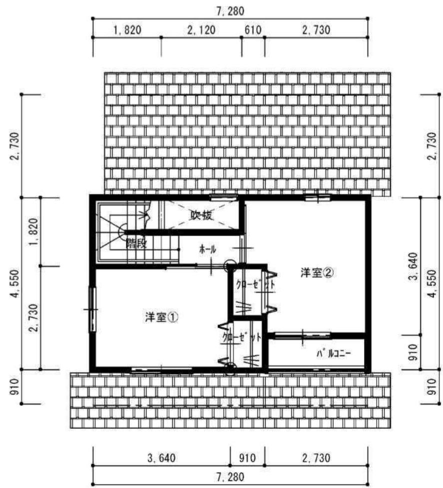
2階平面図
