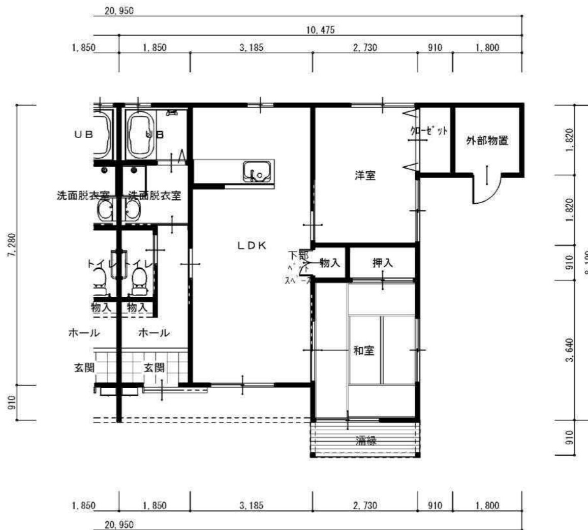
1階 平面図
