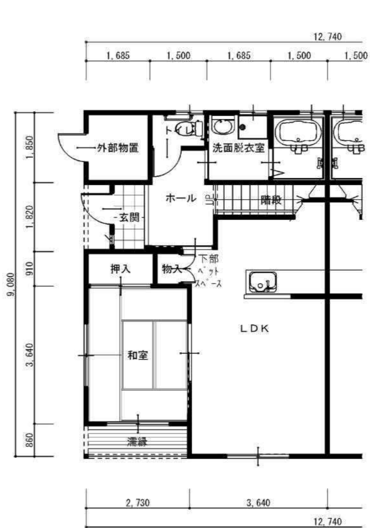
1階 平面図
