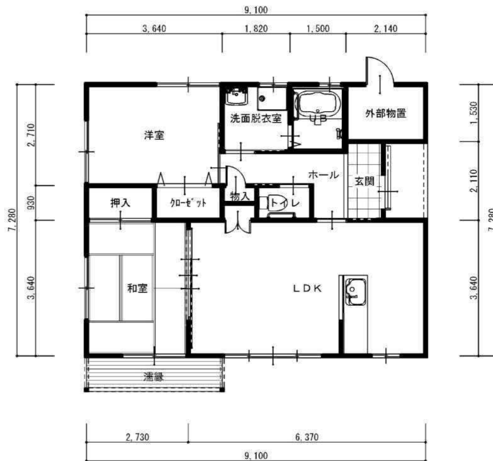
1階 平面図
