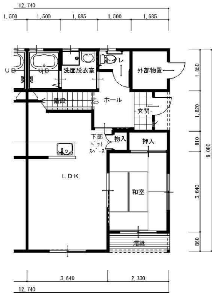
1階 平面図
