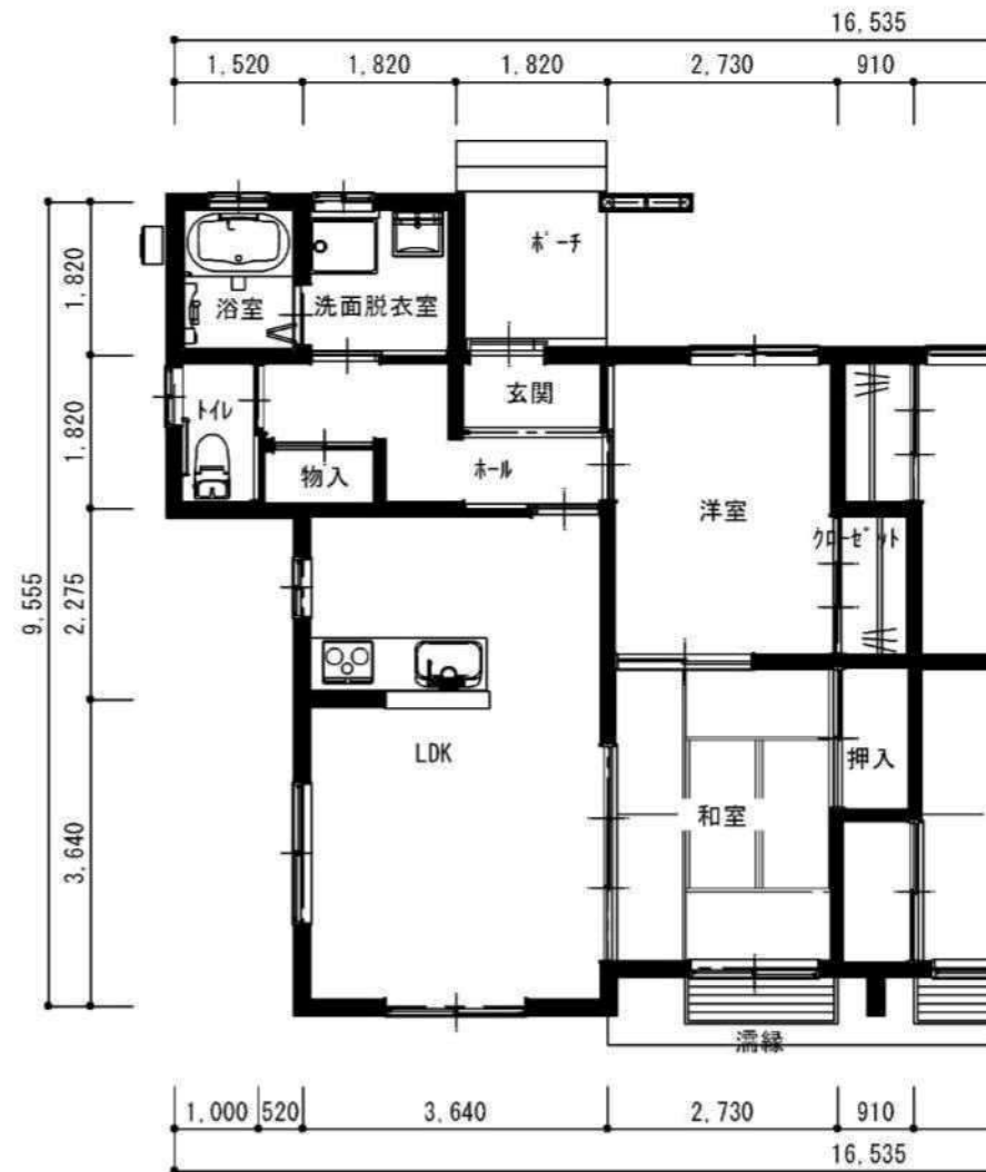
1階平面図
