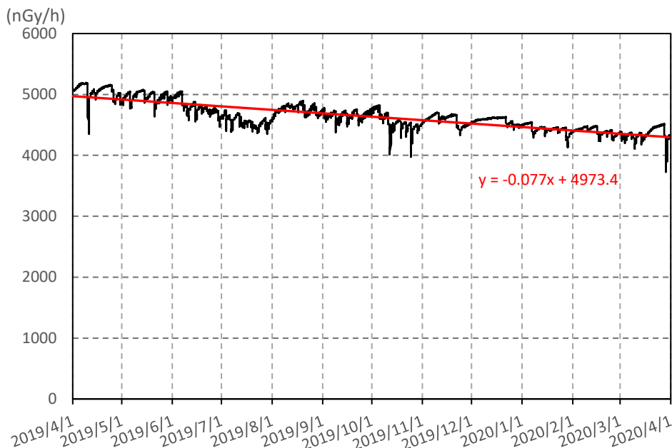
図1 空間線量率（大熊町南台、2019年度）
