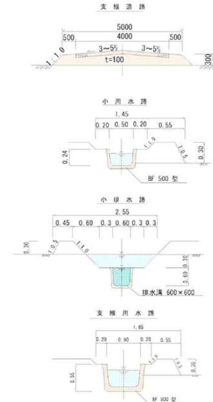
標準構造図
