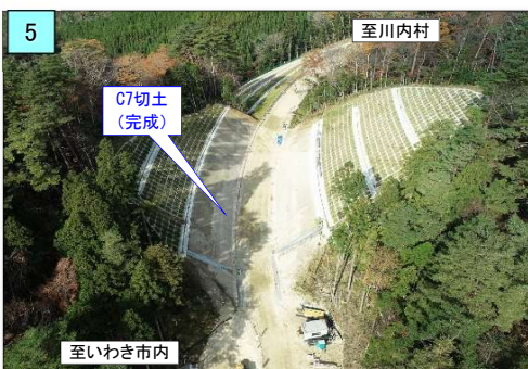
C7切土も最後の段まで掘削完了しました。
