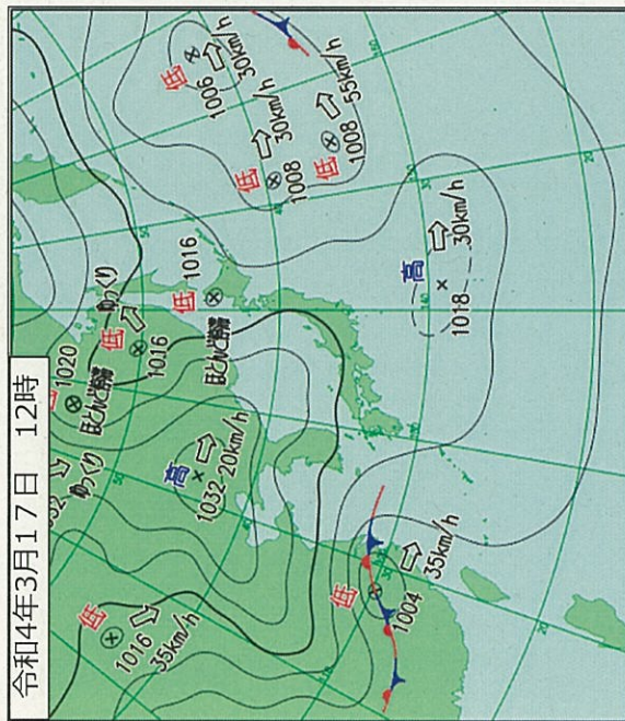
実況天気図 (17日12時)
