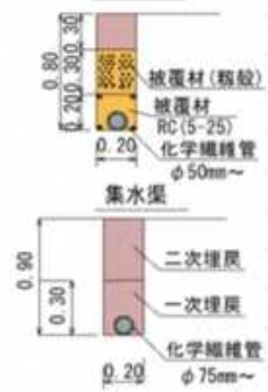
吸水渠
