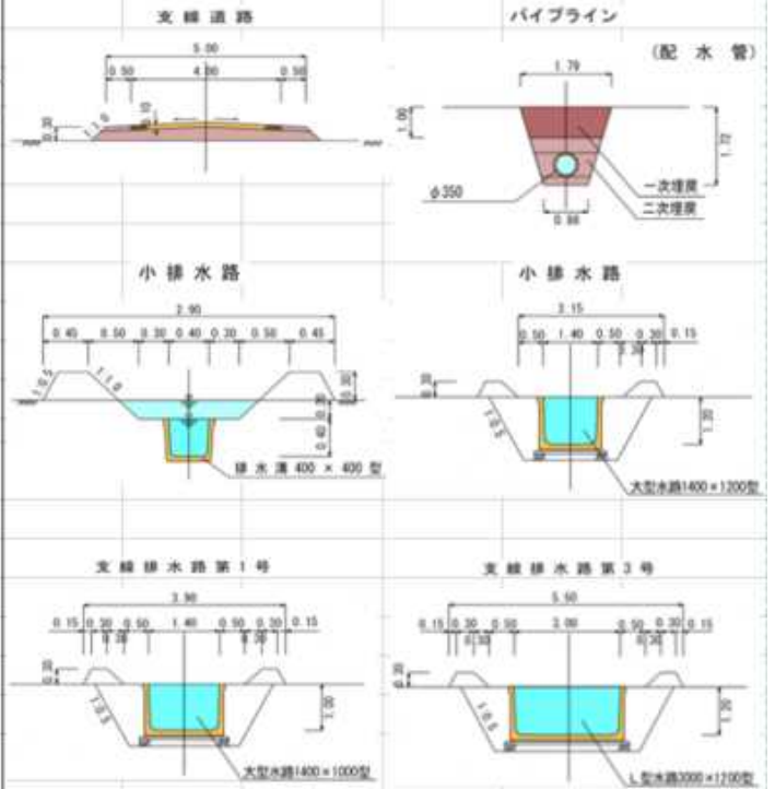
標準構造図
