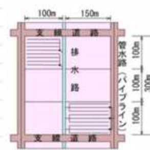
標準区画割図
