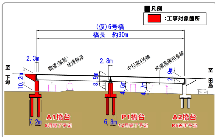
【(仮)6号橋概略図 (側面図)】
