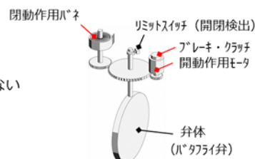
緊急遮断弁-1の構造概略
