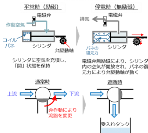
緊急遮断弁-1の構造概略
