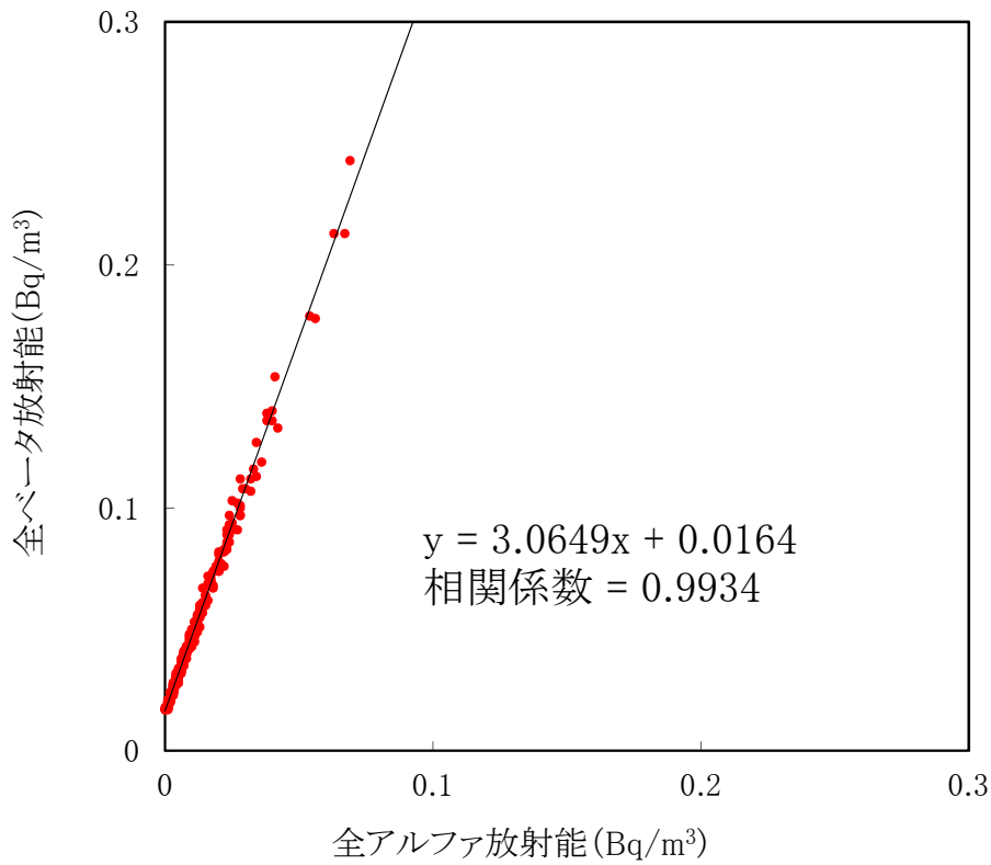
大気浮遊じんの全アルファ・全ベータ放射能の相関図 (MP-1) (令和4年4月～令和4年6月)
