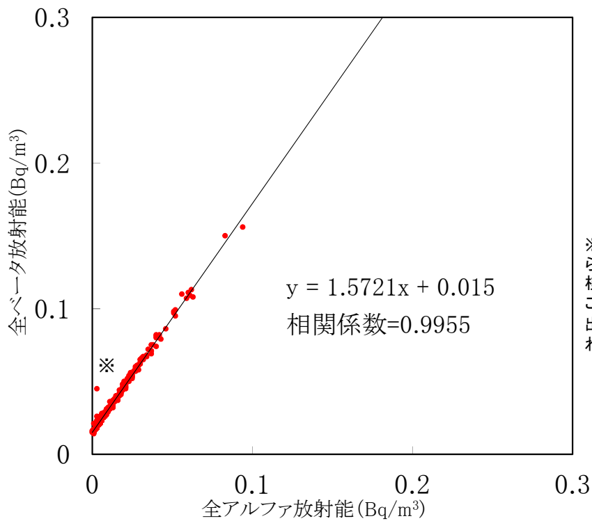
大気浮遊じんの全アルファ・全ベータ放射能の相関図 (MP-8) (令和4年4月～令和4年6月)
