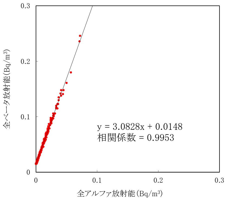
大気浮遊じんの全アルファ・全ベータ放射能の相関図 (MP-7) (令和4年4月～令和4年6月)
