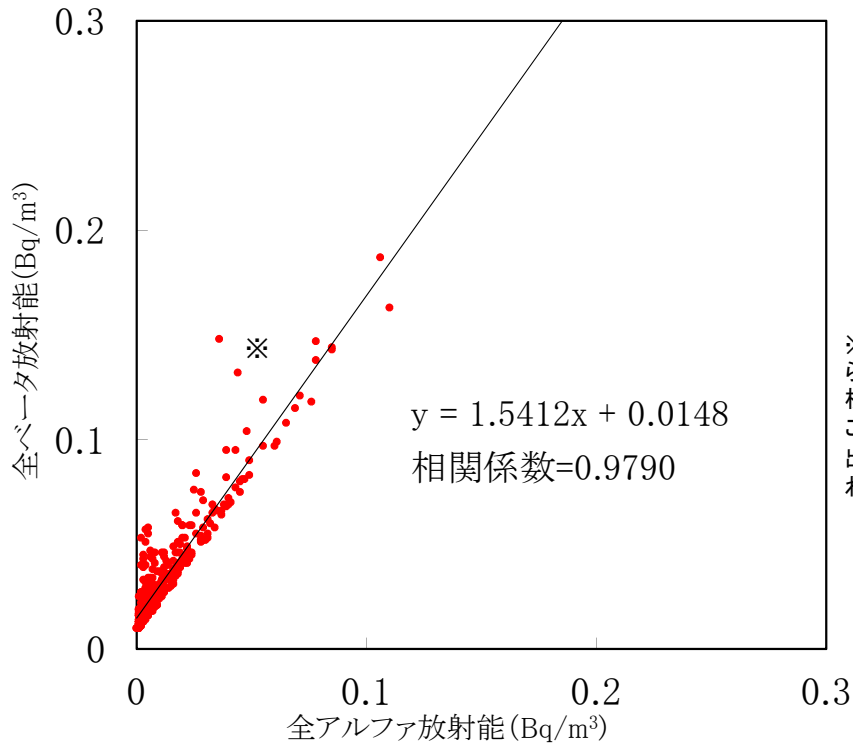
大気浮遊じんの全アルファ・全ベータ放射能の相関図 (MP-3) (令和4年4月～令和4年6月)
