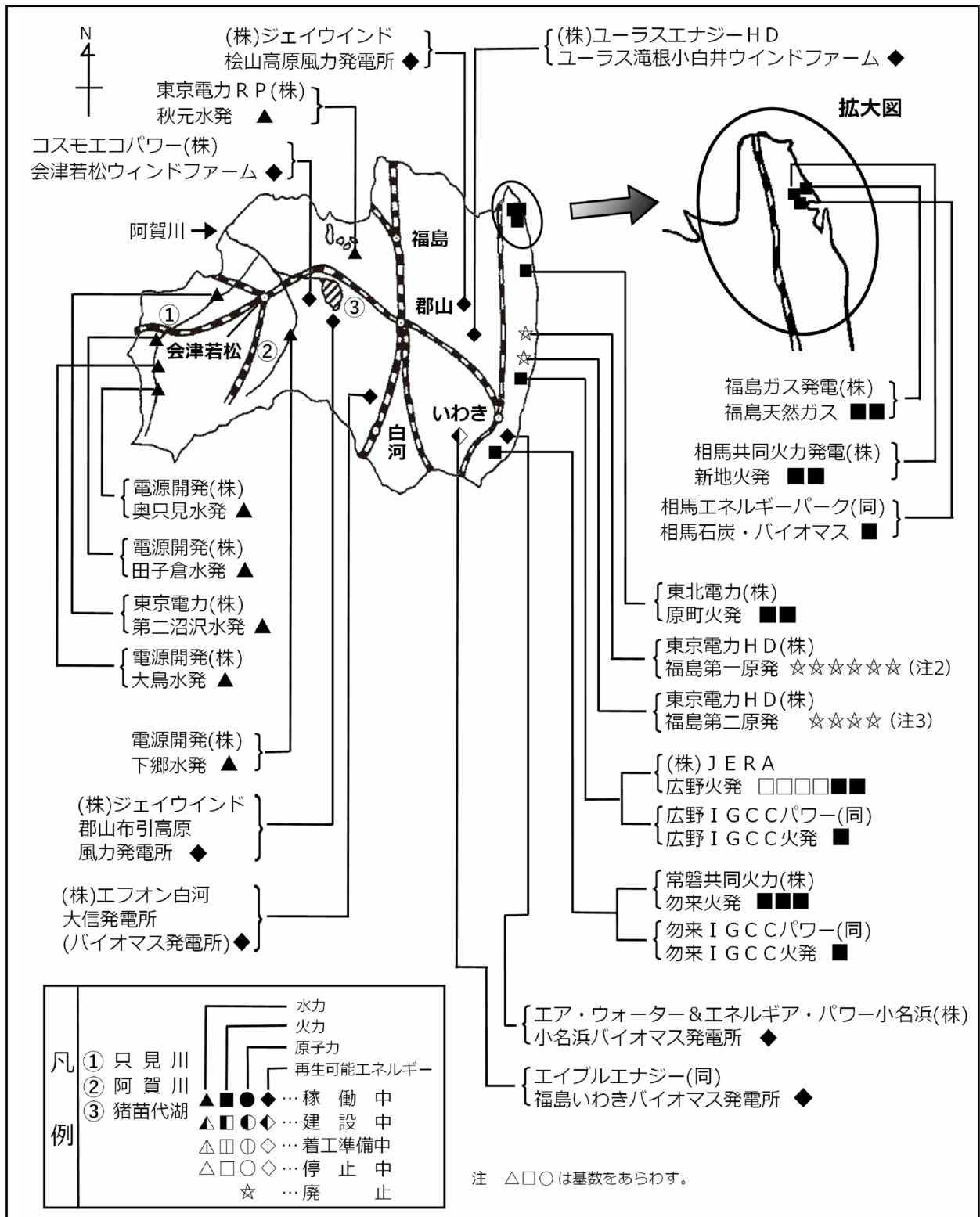
36図 電源立地状況(令和4年7月31日現在)
