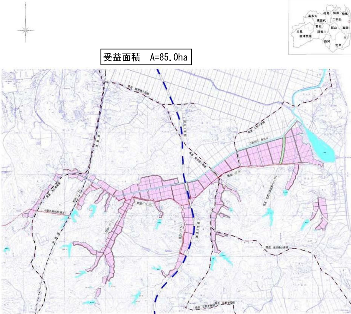
計画一般図
