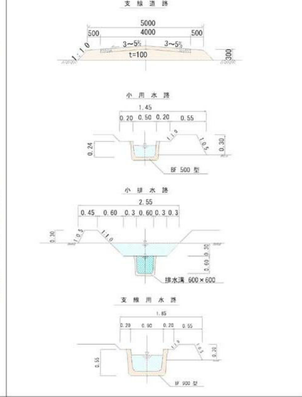
標準構造図
