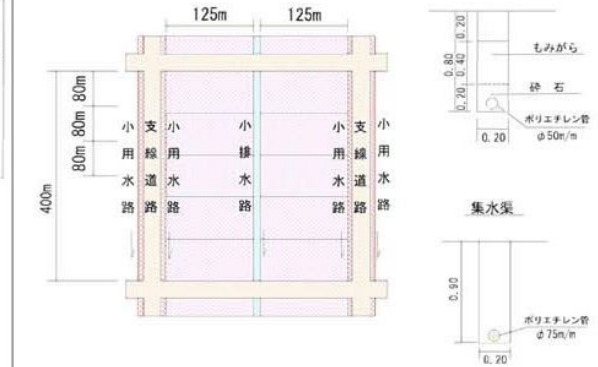
標準構造図
