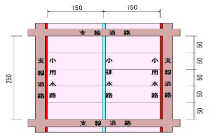
標準構造図
