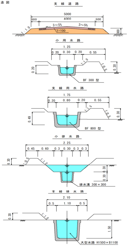
標準構造図
