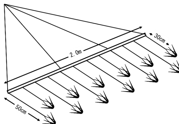
図2 文鎮こぎの構造
