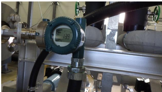
(写真2-1) 圧力計の状況 (清掃前、13.9 kPa)
