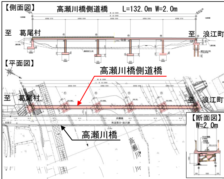
高瀬川橋側道橋
