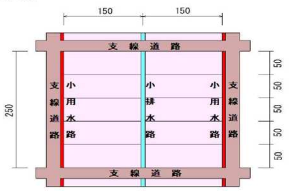
標準構造図
