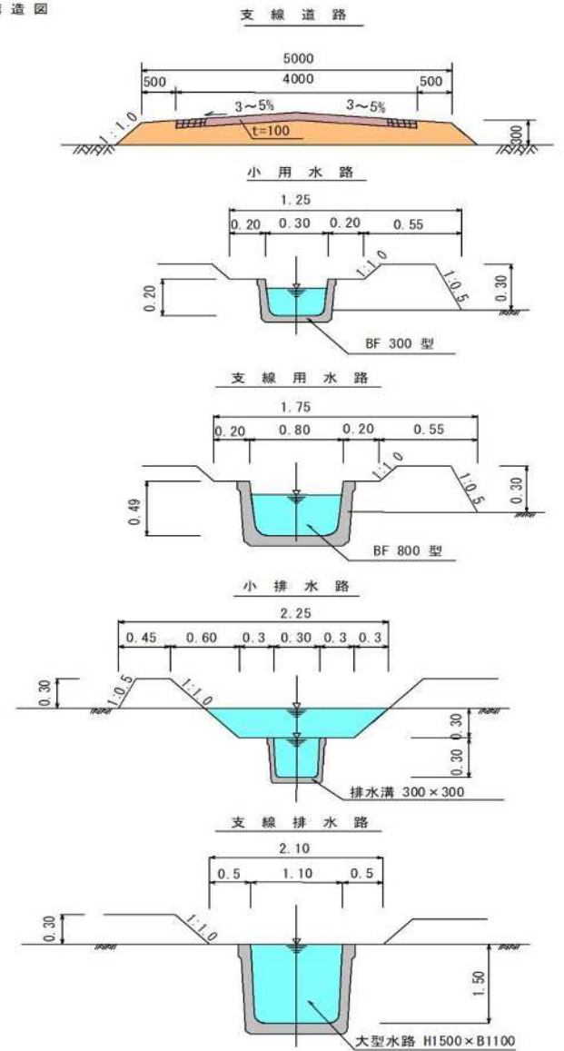
標準構造図
