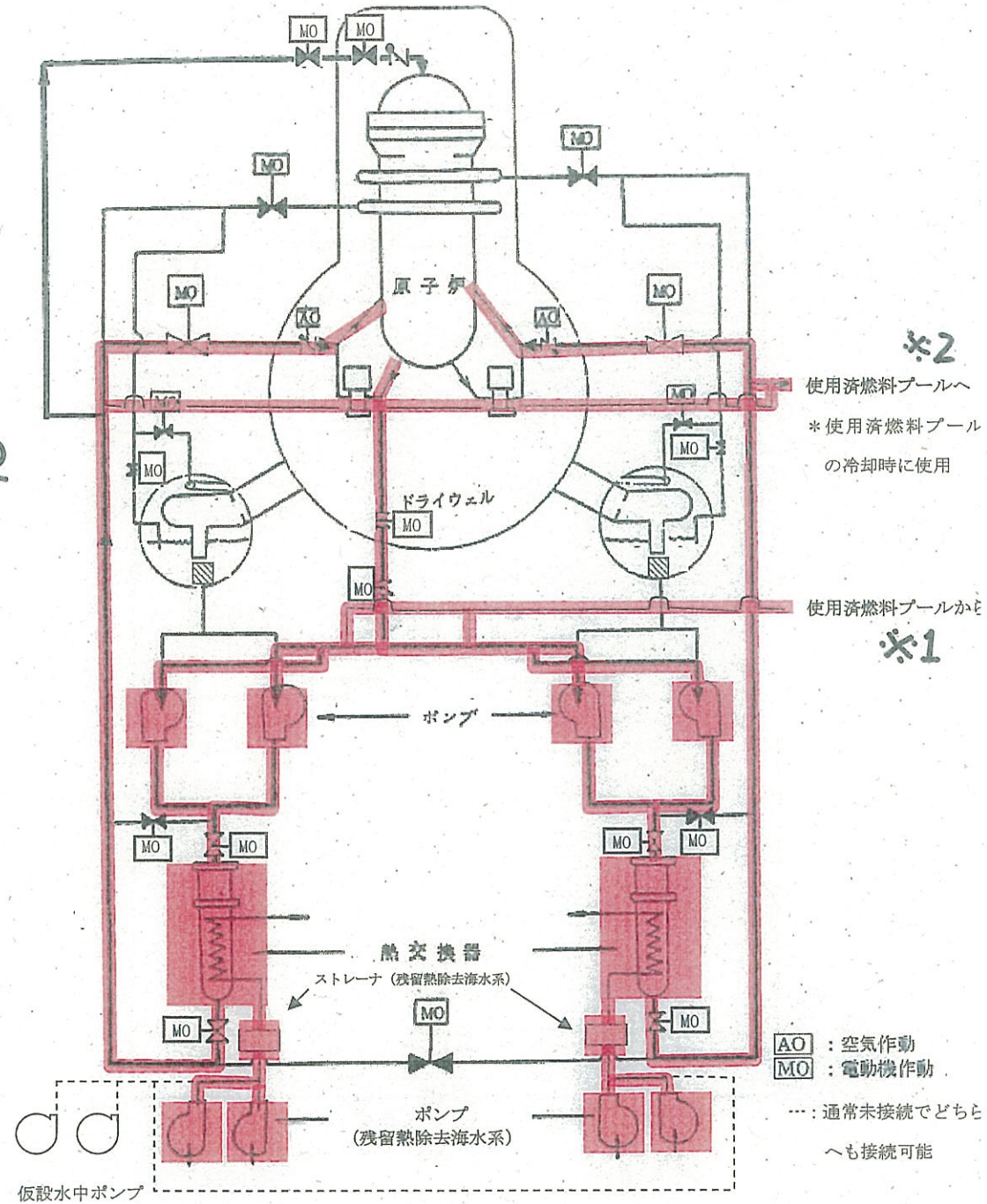
非常時熱負荷運転 (残留熱除去系による使用済燃料プール冷却) 概略図
