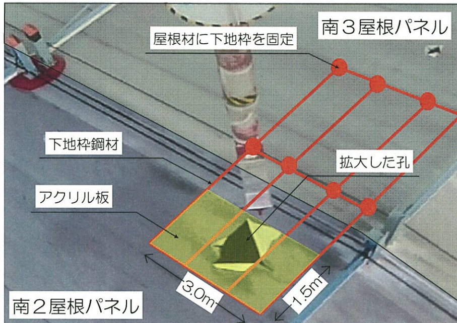
概念図（平面）
