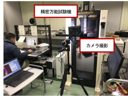
図3 測定機器
