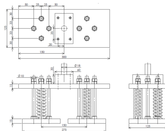
図4 圧縮試験に使用した治具
