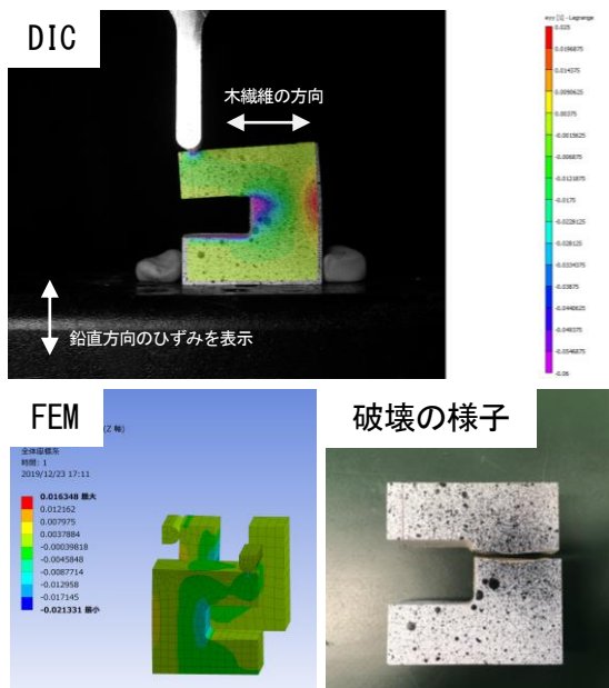
図6 木繊維が水平方向の場合の試験結果
