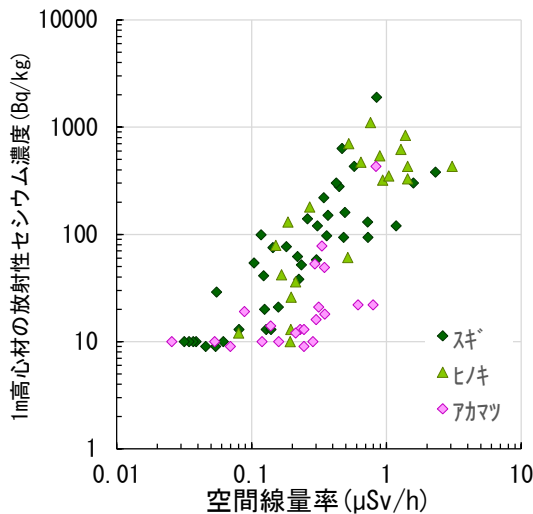
【1m高 心材】
