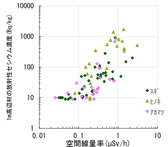
【1m高 辺材】
