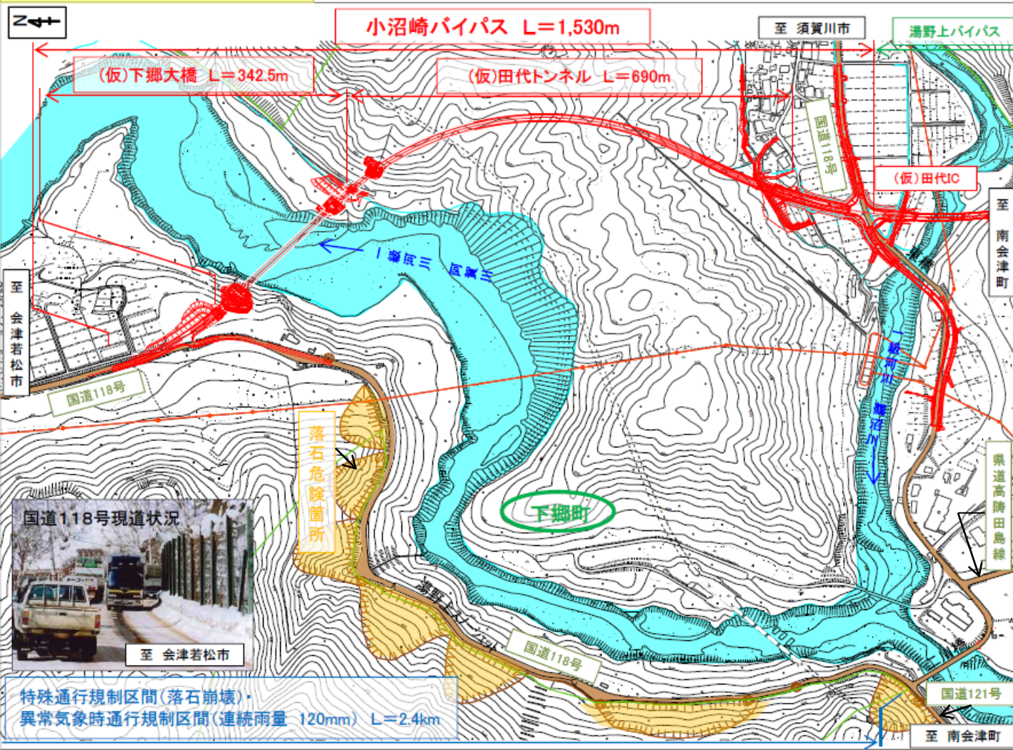
小沼崎バイパス全体平面図
