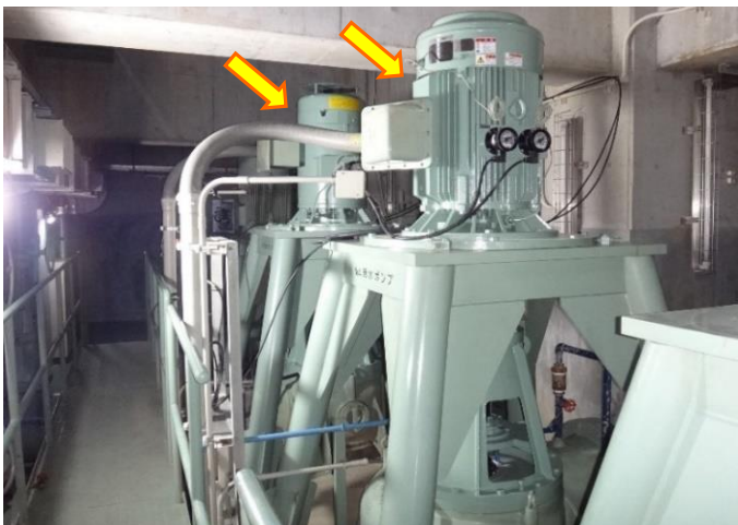
第1スクリーンポンプ棟主ポンプ （左岸幹線の下水を揚水するポンプ）
